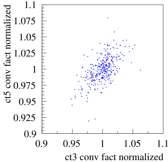
Abbildung 3.5: Korrelation der Konversionsfaktoren innerhalb einer Beobachtungsperiode am Beispiel des Vergleichs von CT 3 und CT 5. Jeder Punkt gibt den Konversionsfaktor q_{el} an, der aus einem für beide Teleskope zeitgleichen Laser-Run bestimmt wurde. Die Werte wurden für jedes Teleskop auf den jeweiligen Periodenmittelwert normiert, um den allgemeinen Alterungseffekt zu unterdrücken. Es gehen Daten von etwas über einem Jahr ein. Man erkennt, daß die Werte für jedes Teleskop eine Reproduzierbarkeit von wenigen Prozent haben, und daß die Streuung der Ergebnisse innerhalb einer Meßperiode durch einen alle Teleskope gemeinsam betreffenden Effekt verursacht sein muß.
