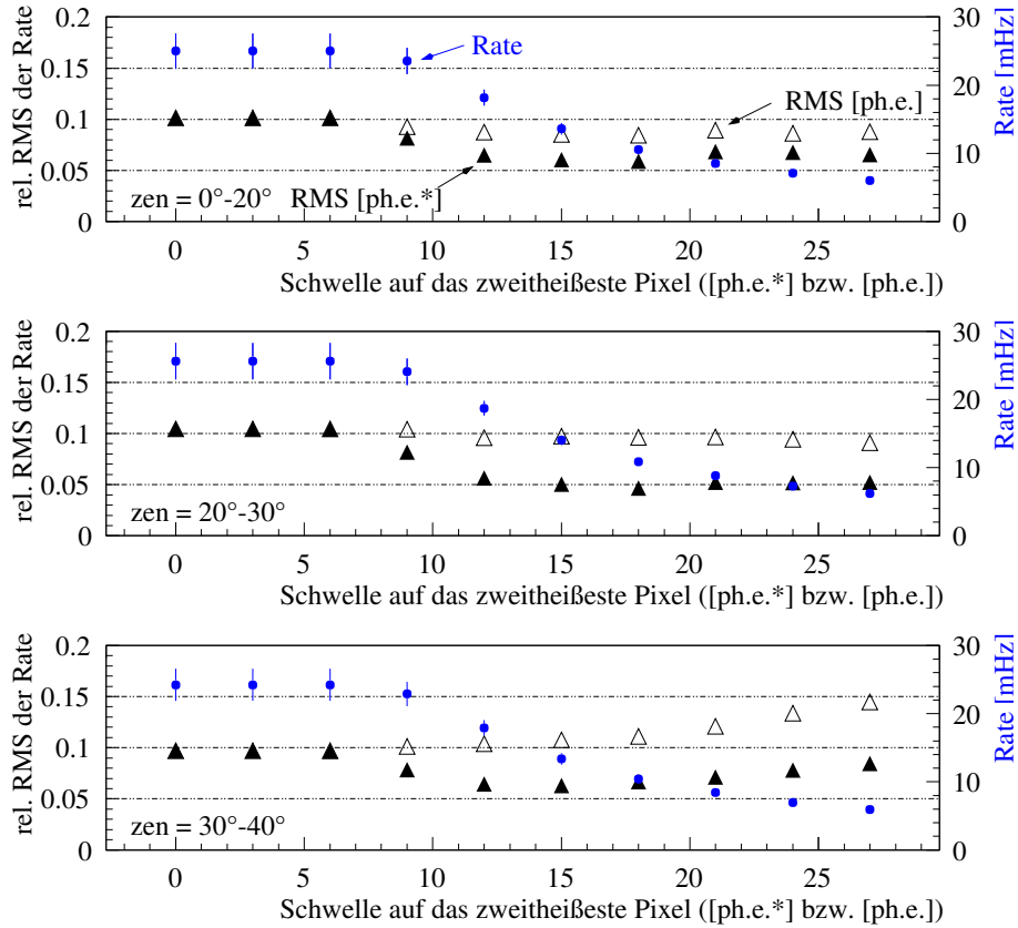
Abbildung 3.10: Bestimmung der minimalen Softwareschwelle, die benötigt wird, um eine möglichst homogene Akzeptanz des Detektors über die volle Laufzeit zu erzeugen. Die gefüllten Dreiecke zeigen die relativen Streuungen der im monatlichen Mittel bestimmten Untergrundraten nach einer Softwareschwelle an, die den Hardwaretrigger auf einer energiegeeichten Amplitudenskala simuliert. Die Streuung wird ab einer Schwelle von 12 ph.e.* minimal. Die offenen Dreiecke zeigen den Effekt derselben Softwareschwelle auf der „rohen“, nicht energiegeeichten Skala an; die Streuung wird erwartungsgemäß nur geringfügig kleiner.
