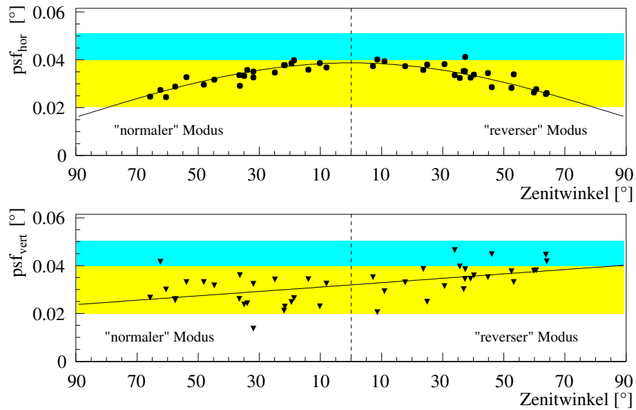
Abbildung 4.11: Dynamische Aufweitung der PSF als Funktion des Zenitwinkels am Beispiel von CT 6 in der Periode 9/98. Oben: Breite der PSF in horizontaler Richtung. Unten: Breite der PSF in vertikaler Richtung. Die Spiegel werden unter 90° Zenitwinkel im normalen Modus justiert, dort ist die optimale PSF zu erwarten und auch zu sehen.
