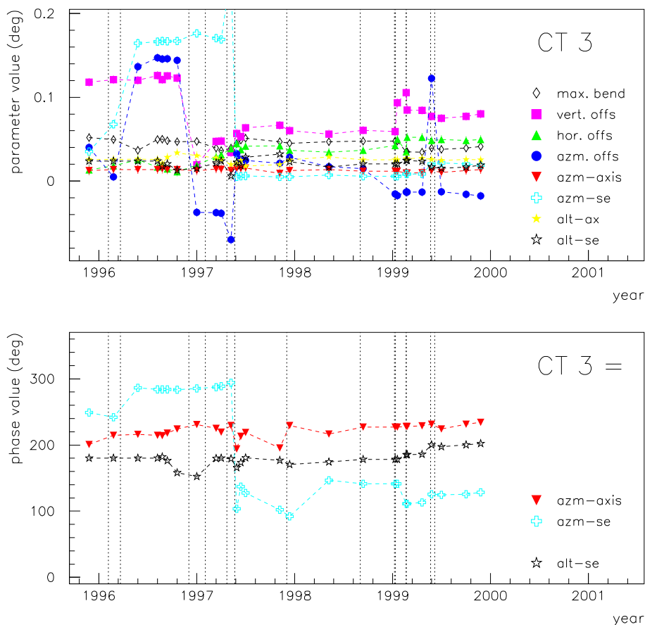
Abbildung 4.9: Die zeitliche „Entwicklung“ der Ausrichtungsparameter, am Beispiel von CT 3. Oben sind Offsets und Amplituden gezeigt, unten die evtl. dazugehörigen Phasen. Die vertikalen gepunkteten Linien geben die Zeitpunkte an, an denen jeweils neue Parametersätze gültig wurden. Falls keine mechanischen Arbeiten zusätzlich die Rekalibration einzelner oder aller Parameter nötig machten, wurde etwa ein- bis zweimal pro Jahr eine vollständige Kalibration durchgeführt, die die Überprüfung aller Parameter ermöglicht. Analoge Verläufe existieren für CT 2 und CT 4-6. Das Bild kann nicht dazu dienen, genaue Informationen über einzelne Parameter zu liefern, sondern soll nur einen Eindruck vom typischen zeitlichen Ablauf geben.
