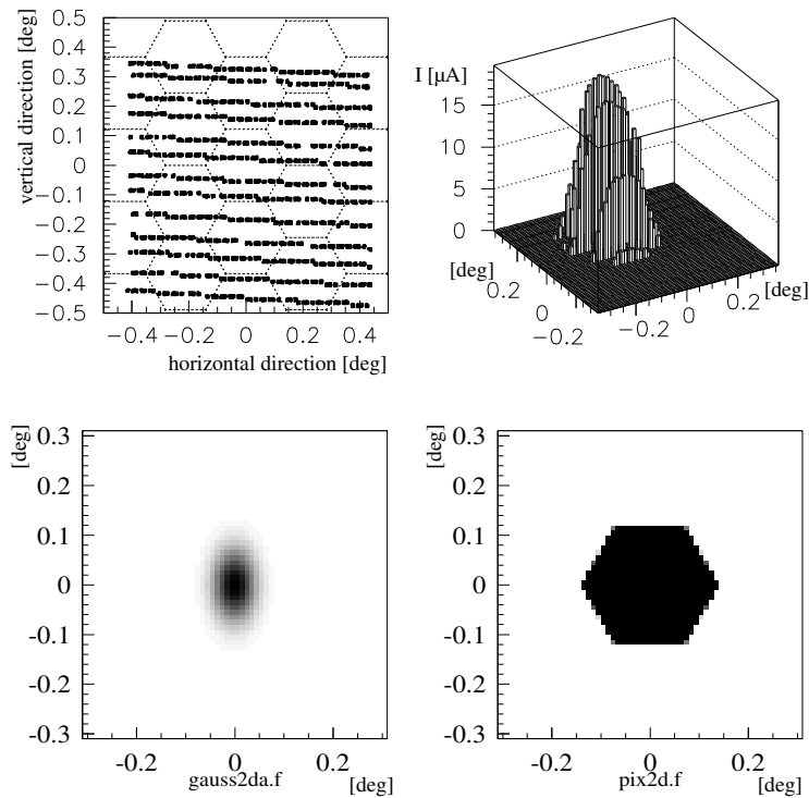
Abbildung 4.1: Prinzip eines Point Runs . Oben links: Sollpositionen des Sterns in der Kameraebene. Das Teleskop fährt horizontale Scan-Linien; da sich der Stern während der Dauer einer Scan-Linie (ca. 30-60 sec) bewegt, sind die Scan-Linien in Bezug auf das Kamerakoordinatensystem leicht geneigt. Oben rechts: Strom im zentralen Pixel als Funktion der Differenz zwischen erwarteter Sternposition und Pixelmittelpunkt. Der Verlauf der Funktion entsteht aus einer Faltung der Pixeloberfläche (unten rechts) und des Sternabbildes in der Kameraebene (unten links); letzteres ist durch die Punktabbildungsfunktion des Reflektors gegeben. Die Pixeloberflächenfunktion wird in guter Näherung einfach durch die geometrische Begrenzung der Lichttrichter definiert (siehe Kap. 2.3.2, Abb. 2.4). Der Abstand zwischen dem Schwerpunkt der Verteilung und dem Koordinatennullpunkt wird durch den Ausrichtungsfehler des Teleskops in der momentanen Position verursacht. Durch eine Rückfaltung der Verteilung mit der Pixeloberflächenfunktion erhält man prinzipiell die Punktabbildungsfunktion des Reflektors in der momentanen Teleskopposition.
