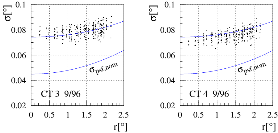
Abbildung 4.5: Bestimmung einer Parametrisierung der PSF . Die Punkte zeigen die Breite der gefitteten zweidimensionalen Gaußfunktion für jedes Pixel. Die untere Funktion gibt die gewonnene Parametrisierung für \sigma_{\text{psf}} an, die obere Funktion die sich daraus ergebenden Erwartungswerte für die Breite der mit der Pixeloberfläche gefalteten Funktion.
