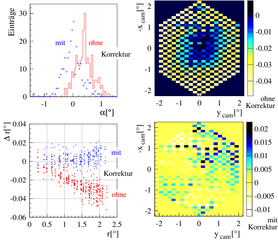
Abbildung 4.4: Analyse eines Full Camera Point Runs im Hinblick auf die Winkelabbildungseigenschaften am Beispiel von CT3, 9/96. Oben links: Werte für \alpha für alle Pixel, ohne und mit Korrektur. Unten links: radiale Abweichung \Delta r von der durch die Winkelabbildung mit f_{nom} = 4.92 m erwarteten Position. Oben rechts: die unkorrigierten Werte von \Delta r in der Kameraebene. Unten rechts: die korrigierten Werte von \Delta r ; im Rahmen der Fehler sind keine Strukturen mehr erkennbar, die z.B. auf eine Verkippung der Kameraebene gegen die Fokalebene hindeuten würden.
