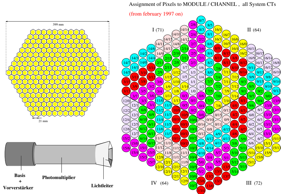
Abbildung 2.4: Links oben: Das Layout der aus 271 Pixeln bestehenden Kameras. Die schattierten Kreise kennzeichnen die Öffnungsfenster der Photomultiplier. Links unten: Ein „Pixel“ besteht aus Lichtleiter ( Funnel ), Photomultiplier, HV-Versorgung (Basis) und Vorverstärker. Rechts: Die Ausleseelektronik ist in VME-Module aufgeteilt, die jeweils 16 Pixel umfassen. Diese Gruppen sind in der Kamera ebenfalls benachbart, was im Bild durch die unterschiedlichen Grautöne angedeutet wird. Dieses Layout führt zu einer gewissen Inhomogenität des Kameragesichtsfeldes (siehe Kap. 8.3.1).
