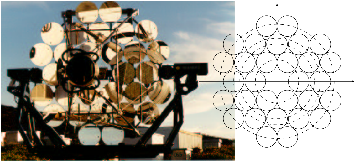
Abbildung 4.2: Spiegellayout der HEGRA-Systemteleskope. Die 30 Einzelspiegel sind auf vier konzentrischen Kreisen angeordnet. Diese entsprechen den in Abb. 4.3, unten, angedeuteten „Ringen“.
