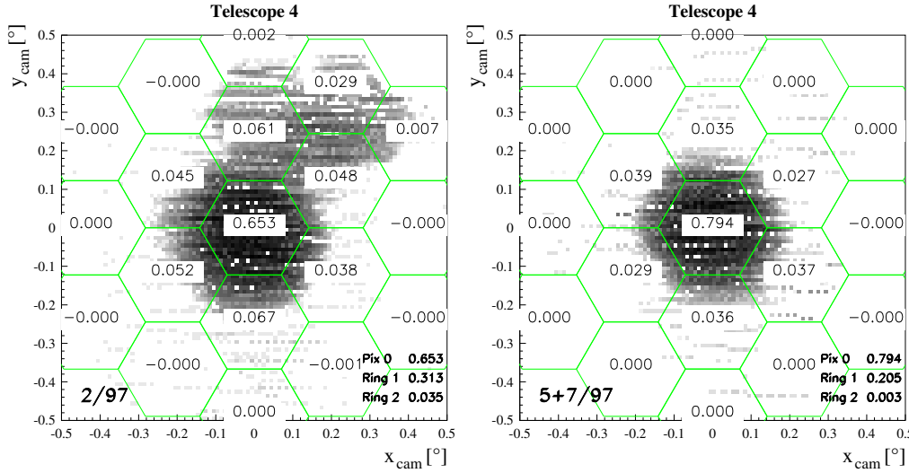
Abbildung 4.10: Einfluß dejustierter Spiegel auf die PSF . Links: Fünf stark dejustierte Spiegel (und eine im Mittel nicht optimale Justierung aller weiteren Spiegel) führen dazu, daß bei gleichmäßiger Ausleuchtung eines Pixels 35% des Lichts in benachbarte Pixel fällt. Rechts: Dasselbe Teleskop nach der Korrektur der Spiegeljustierung. Im Idealfall wird nur 20% des Lichts in die benachbarten Pixel gestreut.
