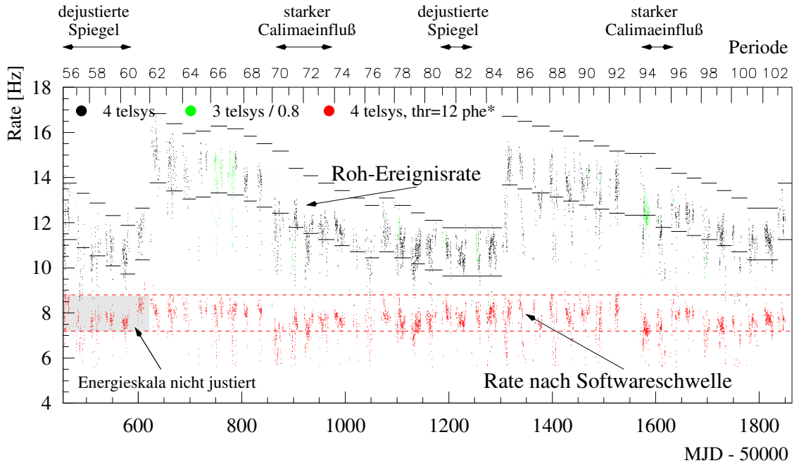
Abbildung 3.8: Ereignisrate des HEGRA-Teleskopsystems. Jeder Punkt stellt die Ereignisrate eines Runs dar; für die Untersuchung wurden nur Runs zugelassen, die unter einem Zenitwinkel von weniger als 30^\circ aufgenommen wurden. Das obere Band stellt die Roh-Ereignisrate dar; diese ist im wesentlichen mit der Systemtriggerrate identisch und ein Maß für die Empfindlichkeit des Systems. Aus dieser Ratenverteilung wurde eine monatliche „Soll“-Ereignisrate bestimmt; die Begrenzungsmarkierungen kennzeichnen die Rate, die \pm 10\% von dieser nominellen Rate abweicht. Die jeweiligen Ausläufer in der Verteilung zu niedrigen Raten werden dominant durch Runs bedingt, die unter reduzierten Wetterbedingungen aufgenommen wurden. Das untere Band stellt die Ereignisrate derselben Runs nach Anwendung einer Softwareschwelle dar, die dazu dient, nachträglich eine zeitlich konstante Akzeptanz des Systems zu erzeugen. Man erkennt, daß dies innerhalb des wiederum 10-prozentigen Fehlerbandes gut gelingt (weitere Details siehe Text). Um das Bild zu säubern und die klare Darstellung der beiden Ereignisraten zu ermöglichen, wurden ausschließlich für die Abbildung alle Runs verworfen, die mehr als 30% von der jeweiligen nominellen Ereignisrate abweichen. Der Plot beginnt mit dem Januar 1997 und reicht bis November 2000.
