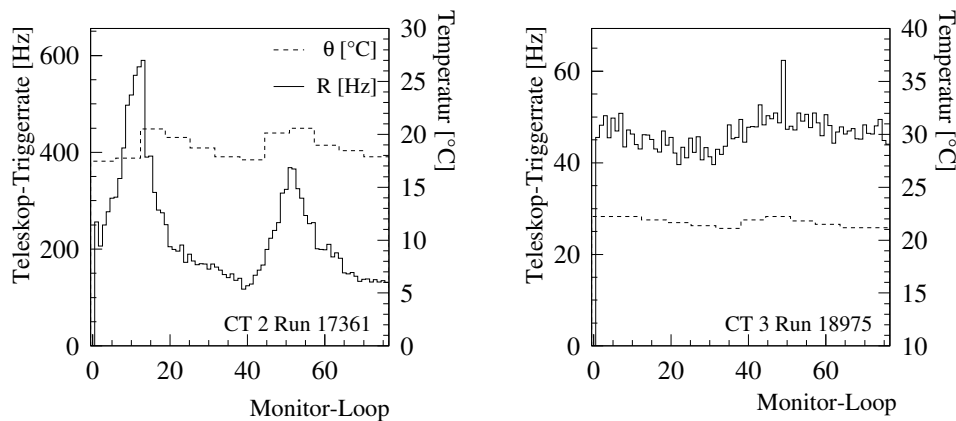
Abbildung 3.2: Änderung der Einzelteleskop-Triggerrate im Verlauf eines Runs, zusammen mit der an der Ausleseelektronik gemessenen Temperatur. Ein Monitor-Loop dauert 16 Sekunden. Der Temperaturverlauf wird durch den etwa 10-minütigen Zyklus der Klimaanlage in den Elektronikcontainern verursacht. Man erkennt die klare Korrelation zwischen Rate und Temperatur, die bei CT 2 am stärksten ausgeprägt ist; bei allen weiteren Teleskopen liegt die Streuung bei 20-40%. Ursache ist vermutlich eine temperaturabhängige Änderung der Ansprechwahrscheinlichkeit der Diskriminatoren; eine Änderung im Rauschverhalten ist ebenfalls denkbar. Eine Änderung der Verstärkung in dieser Größenordnung erscheint sehr unwahrscheinlich. Beispiel eines typischen Hardware Check -Histogramms.
