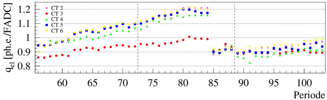
Abbildung 3.7: Die zeitliche Entwicklung der elektrischen Konversionsfaktoren q_{el} von 1997 bis 2000. Bis einschließlich Periode 72 wurde in der Pulsformanalyse ein konstanter Wert von 1 für alle Teleskope angenommen, seit Periode 73 gehen die Meßwerte in die Berechnung der Pixelamplituden ein. Am Beginn von Periode 85 wurde die Hochspannung aller Pixel in allen Teleskopen angehoben, um den vorausgegangenen Effizienzverlust auszugleichen. Seit Periode 89 wird in der Analyse der korrigierte Wert für den Phasenfehler angewendet. Da die Laser eine typische Amplitude von 50-100 Photoelektronen pro Blitz erzeugen, wurde der Konversionsfaktor bis dahin um ca. 6% zu groß berechnet (siehe Abb. 3.6). Die Abbildung zeigt die in der Datenaufbereitung ab Periode 73 tatsächlich verwendeten Zahlen; in Abb. 3.9, Mitte, ist die daraus abgeleitete Verstärkungsänderung gezeigt, die um den 6%igen Fehler korrigiert ist.
