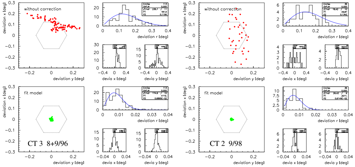
Abbildung 4.8: Die aus den Point Runs ermittelten Verschiebungsvektoren in der Kameraebene für die in Abb. 4.7 gezeigten Kalibrationen. Jeder Punkt entspricht einem Point Run . In der oberen Hälfte der Abbildungen sind jeweils die Ergebnisse der Kalibrationsmessungen gezeigt; das Sechseck deutet die Abmessungen des zentralen Pixels an. Unten wurde in der Analyse der Point Runs bereits die Ausrichtungskalibration angewendet. Die verbleibenden Fehlausrichtungen (Residuen) sind ein Maß für die Genauigkeit der Kalibration; sie beträgt 0^{\circ}007 in radialer Richtung bzw. 0^{\circ}005 pro Achse.
