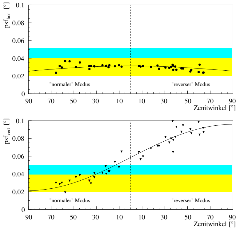
Abbildung 4.13: Die Breite der Punktantwort von CT2 in horizontaler (oben) und vertikaler (unten) Richtung. Die horizontale PSF ist stabiler als bei den anderen Systemteleskopen. Die vertikale PSF hingegen ist deutlich schlechter und in dieser Form über weite Bereiche der Teleskopausrichtung inakzeptabel.
