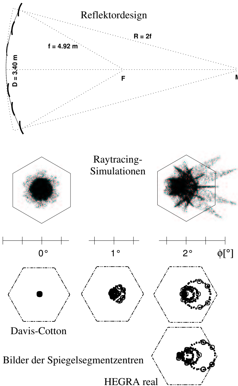
Abbildung 4.3: Oben: Prinzip des Davies-Cotton-Designs. Der Reflektor bildet einen Sphärenabschnitt mit dem Brennpunkt als Mittelpunkt. Die Einzelspiegel sind jedoch wie üblich auf einen Punkt in der Entfernung 2f ausgerichtet. Mitte: Raytracing-Simulationen für die PSF der HEGRA-Reflektoren, auf der optischen Achse und unter einem Einfallswinkel von 2^\circ . Unten: Bilder der Einzelspiegel-Mittelpunkte unter verschiedenen Einfallswinkeln. Die kleinen Punkte würden für eine dichte Bestückung kleiner Segmente gelten; sie bilden Ringe, die einer festen Entfernung der Segmente auf dem Reflektor in Bezug zur optischen Achse entsprechen. Die offenen Kreise spiegeln die reale Bestückung der HEGRA-Reflektoren wieder.
