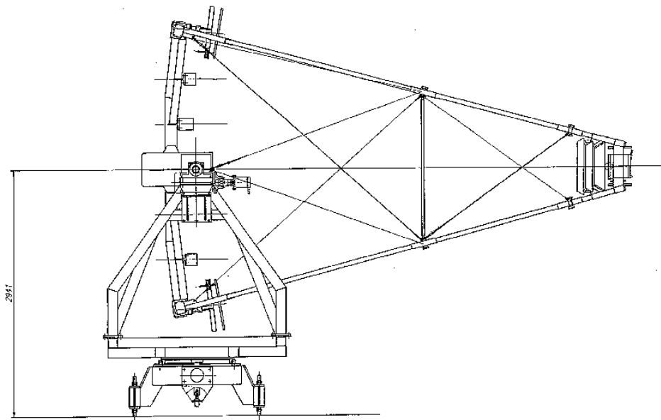
Abbildung 4.6: Technische Zeichnung eines der HEGRA-Systemteleskope. Die Masten bestehen aus leicht flexiblen Kohlefasermasten; die Mastenkonstruktion wird durch Stahlseile versteift.
