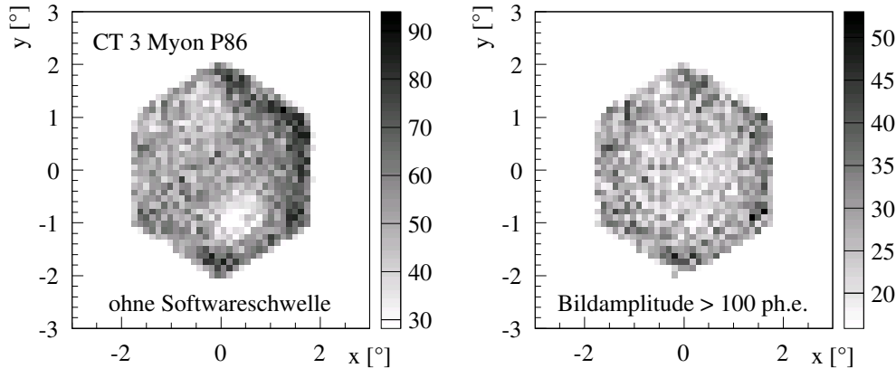
Abbildung 8.2: In Myon-Runs können die Akzeptanzunterschiede der einzelnen Diskriminator-module studiert werden, da hier die Teleskope ausschließlich sich selbst triggern. Die Unterschiede äußern sich in einer Variation der Häufigkeit der rekonstruierten Bildschwerpunkte, die in der Abbildung in Abhängigkeit der Kameragesichtsfeldkoordinaten aufgetragen sind. Ohne Softwareschwelle (links) sind deutliche Akzeptanzunterschiede erkennbar, die nach einer Softwareschwelle auf die Bildamplituden (rechts) verschwinden; die Häufung der Bilder am Kamerarand ist aufgrund abgeschnittener Bilder normal. Bei normalen Daten-Runs ist die Verteilung der Bildschwerpunkte durch die Geometrieeffekte des Systemtriggers dominiert und sagt unmittelbar nichts mehr über die Ansprechwahrscheinlichkeiten der Kameras aus. Die Akzeptanzunterschiede sind allerdings bei Myon-Runs stärker ausgeprägt als in normalen Daten-Runs, da hier die Pixeltriggerschwelle niedriger liegt (5 mV anstatt 8 mV).
