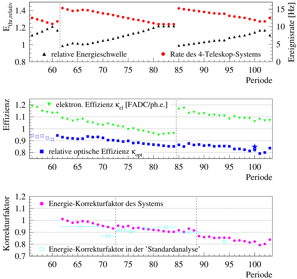
Abbildung 3.9: Energiekalibrationswerte von Januar 1997 bis November 2000. Oben: Nominelle Ereignisrate und relative System-Energieschwelle. Die Energieschwelle liegt bei optimalen Bedingungen bei 500 GeV und im schlechtesten Fall bei 600 GeV. Mitte: Elektronische Effizienz und relative optische Effizienz, die bei der Energieeichung ermittelt wurden. Man erkennt eine Alterung der Photomultiplier von 6% pro Jahr, und einen Reflektivitätsverlust der Spiegel von ca. 3% pro Jahr. Der Sprung in der elektronischen Verstärkung wurde durch eine HV-Anpassung aller Pixel in allen Teleskopen verursacht. Der Stern zeigt den Mittelwert von Reflektivitätsmessungen an einer Reihe von Teleskopspiegeln, relativ zu einem neuen (Referenz-)Spiegel. Unten: Korrekturfaktor, der auf die im DST-Format enthaltenen Bildamplituden angewendet werden muß, um aus ihnen die Schauerenergie berechnen zu können. Zu Details siehe Text.
