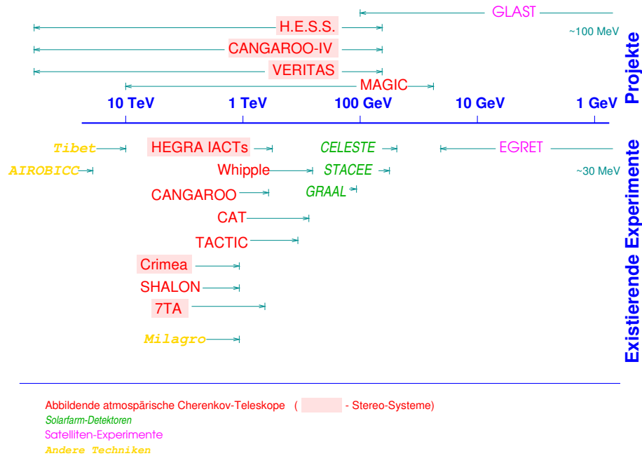
Abbildung 1.4: Übersicht über die zur Zeit in Betrieb befindlichen bzw. geplanten Gamma-Teleskope. Die mit einer Schattierung unterlegten Experimente sind stereoskopische Cherenkov-Teleskop-Systeme. Nach [Kon01].
