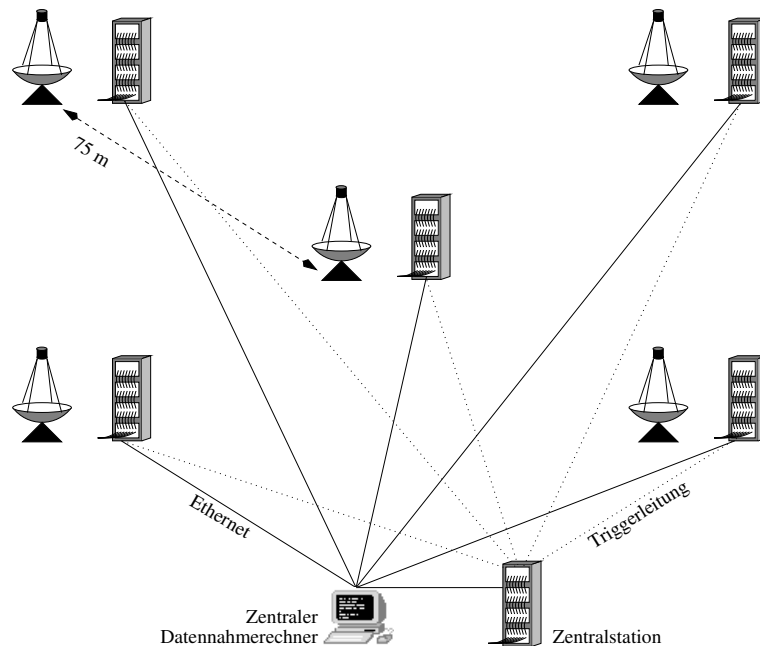
Abbildung 3.1: Signalwege des HEGRA-Teleskopsystems. Die gepunkteten Linien stellen Triggerleitungen, die durchgezogenen Linien Ethernet-Datenverbindungen dar. Die Zentralstation und der zentrale Datennahmerechner befinden sich beide in unmittelbarer Nähe des zentralen Teleskops (CT 3).
