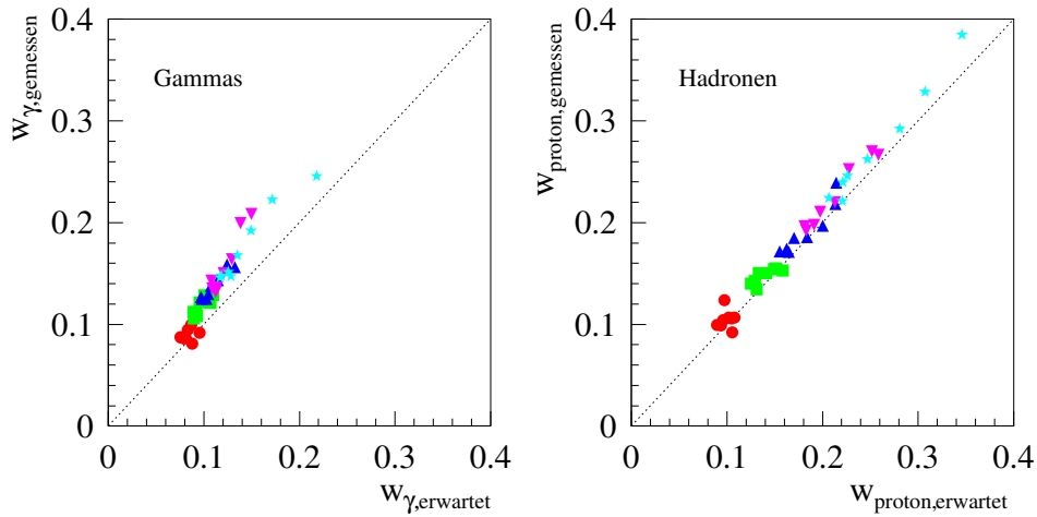
Abbildung 7.5: Vergleich der Width -Erwartungswerte zwischen einer Periode mit schlechter Spiegeljustierung (CT 4, Perioden 58-60) und normaler Spiegeljustierung. Links ist der Vergleich für \gamma 's, rechts für Untergrundereignisse gezeigt. Die Tabellen wurden in beiden Fällen aus Daten erzeugt, die mit Standard-Tail Cuts (3/6 ph.e.) produziert worden sind.
