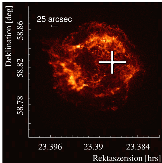
Abbildung 6.2: Schwerpunkt der TeV- \gamma -Emission von Cas A in J2000-Koordinaten. Der systematische Ausrichtungsfehler des HEGRA-Teleskopsystems beträgt 25'' . Zum Vergleich ist das hochaufgelöste Chandra-Röntgenbild bei 0.1 – 10 keV (mit freundlicher Genehmigung von NASA/CXC/SAO) untergelegt; der Mittelpunkt wurde auf die J2000-Koordinaten gelegt.
