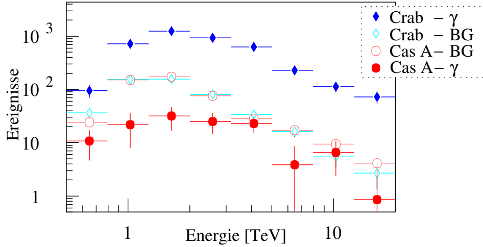
Abbildung 10.7: Rohspektren des Cas A- und des Krebsnebel-Datensatzes (Zenitwinkel 25^\circ - 40^\circ ) im Vergleich. Für alle Daten gelten harte Schnitte ( 0.5 < msw < 1.1 , \theta^2 < 0.0135^\circ^2 ). Die Untergrunddaten werden aus Kontrollregionen gewonnen, deren Fläche im Gesichtsfeld siebenmal größer ist als die Fläche der Signalregion. Die Krebsnebel-Daten sind entsprechend der unterschiedlichen Beobachtungszeiten hochskaliert.
