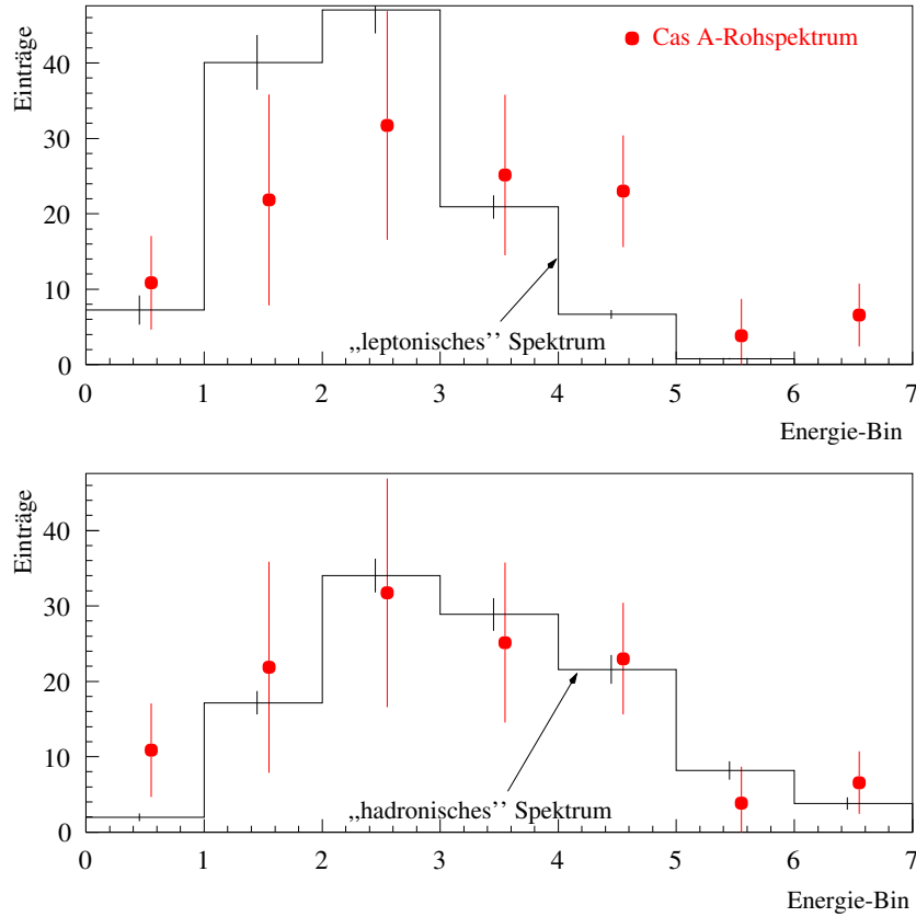
Abbildung 10.10: Vergleich des Cas A- \gamma -Rohspektrums mit einem „leptonischen“ (oben) und einem „hadronischen“ (unten) Modellspektrum. Die Modellspektren wurden aus den Krebsnebel- \gamma -Rohspektrern unter Anwendung der spektralen Verläufe der theoretischen Vorhersagen gewonnen. Für die Normalisierung der Modellspektren in der Darstellung wurde die beste \chi^2 -Anpassung gewählt.
