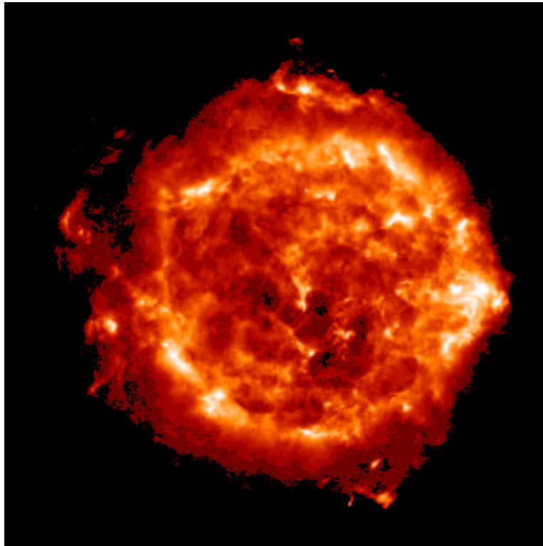
Abbildung 11.1: Radiobild von Cassiopeia A bei 6.3 cm [Tuf86]. Als dominante Strukturen treten der sogenannte Radioring (dunkel) hervor, der von dem diffusen Plateau (helle Strukturen) umgeben wird. Weiterhin sind kleine Strukturen – die sogenannten Radioknoten – zu erkennen, die sich insbesondere durch eine vergleichsweise breite Streuung der spektralen Indizes der Radioemission auszeichnen. Am äußeren Rand des diffusen Plateaus, nicht sichtbar im Bild, befindet sich die äußere Schockfront, an der dominant Beschleunigung von hochenergetischen Teilchen (Hadronen und Elektronen) stattfinden soll.
