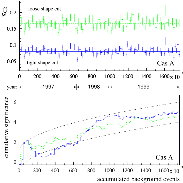
Abbildung 7.11: Verteilungen des Cas A-Datensatzes. Oben: Untergrundunterdrückungseffizienz \kappa_{BG} des harten und des lockeren msw -Schnitts. Unten: Kumulative Signifikanz der Quellmessung nach Anwendung des harten (durchgezogene Linie) und des lockeren (gestrichelte Linie) Schnitts. Die gepunkteten Kurven geben den \pm 1\sigma -Bereich des erwarteten Signifikanzverlaufes an, unter der Annahme einer konstanten \gamma -Emission und eines 5\sigma -Signals am Ende der Messung. Für alle Werte gilt ein Winkelschnitt von \theta^2 < 0.0135^\circ^2 .
