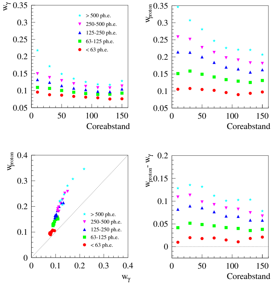
Abbildung 7.1: Width-Erwartungswerte, die aus \gamma - und Untergrundereignissen von Mrk 501-Daten gewonnen wurden. Die Erwartungswerte wurden in dte -Abschnitten von jeweils 20 m und in amp -Bins entsprechend der Formel (\log(amp) - 1.5)/0.3 gewonnen; außerdem wurden nur Daten zwischen 0^\circ und 20^\circ Zenitwinkel verwendet. Oben links: w_\gamma -Erwartungswerte als Funktion des Abstands des Teleskops zum Schauercore für verschiedene Amplitudenbereiche. Oben rechts: Untergrunderwartungswerte in derselben Auftragsung. Unten links: Vergleich der \gamma - und Untergrunderwartungswerte in einer Art Phasendiagramm; auf der Diagonalen liegende Punkt würden eine Übereinstimmung der mittleren Erwartungswerte von \gamma - und Untergrundereignissen bedeuten. Da kleinere Erwartungswerte im Mittel aber auch weniger streuen, sagt der Abstand zur Diagonalen nicht unmittelbar etwas über die Trennschärfe aus. Unten rechts: Differenz der \gamma - und Untergrunderwartungswerte, aufgetragen gegen den Coreabstand. Auch hier gilt die genannte Einschränkung bei der Bewertung der Trennschärfe.
