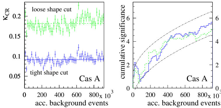
Abbildung 7.12: Dieselben Daten wie in Abb. 7.11, allerdings nach Anwendung der Softwareschwelle zum spektralen Akzeptanzausgleich. Die leichte Verschlechterung der Untergrundunterdrückung des 1999er-Datensatzes ist möglicherweise ein leichtes Indiz für einen verbleibenden Einfluß der im Laufe der Zeit reduzierten optischen Effizienz der Teleskope. Der Effekt ist jedoch (noch) marginal.
