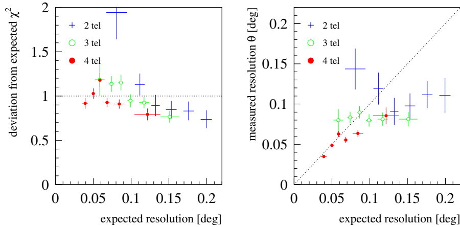
Abbildung 9.10: Für einen mittleren Zenitwinkelbereich ( 20^\circ - 40^\circ ) ist das Ergebnis des \chi^2 -Test und der \theta^2 -Parametrisierung gezeigt. Im Rahmen des statistischen Fehlers stimmen die Ergebnisse in etwa mit den Daten bei kleinen Zenitwinkeln überein.
