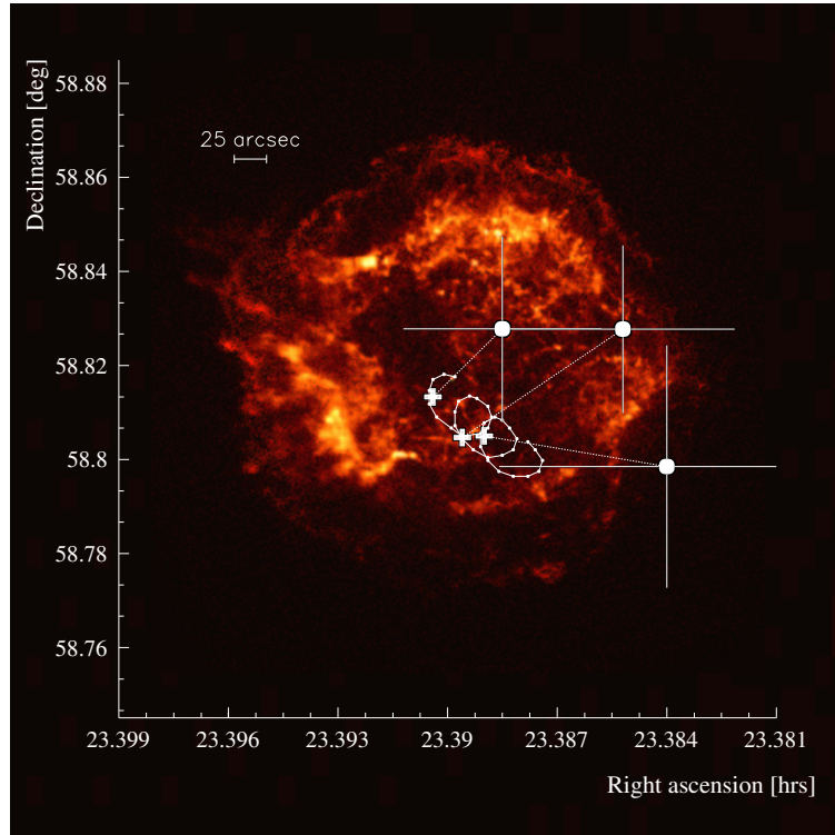
Abbildung 9.4: Die rekonstruierten Schwerpunkte der TeV- \gamma -Emission von Cas A im Vergleich zum Röntgenbild. Die Daten wurden entsprechend der Beobachtungsperioden aufgeteilt. Als Referenz ist das hochaufgelöste Chandra-Röntgenbild bei 0.1 – 10 keV (mit freundlicher Genehmigung von NASA/CXC/SAO) untergelegt; der Mittelpunkt wurde auf die J2000-Koordinaten gelegt. Die durch eine durchgezogene Linie verbundenen Punkte kennzeichnen den Weg dieser Position von 1997 bis 2000, wenn die Korrektur auf eine gemeinsame Epoche unterlassen wird. Die offenen Kreuze kennzeichnen die mittlere erwartete Position des Mittelpunkts von Cas A für die jeweilige Periode.
