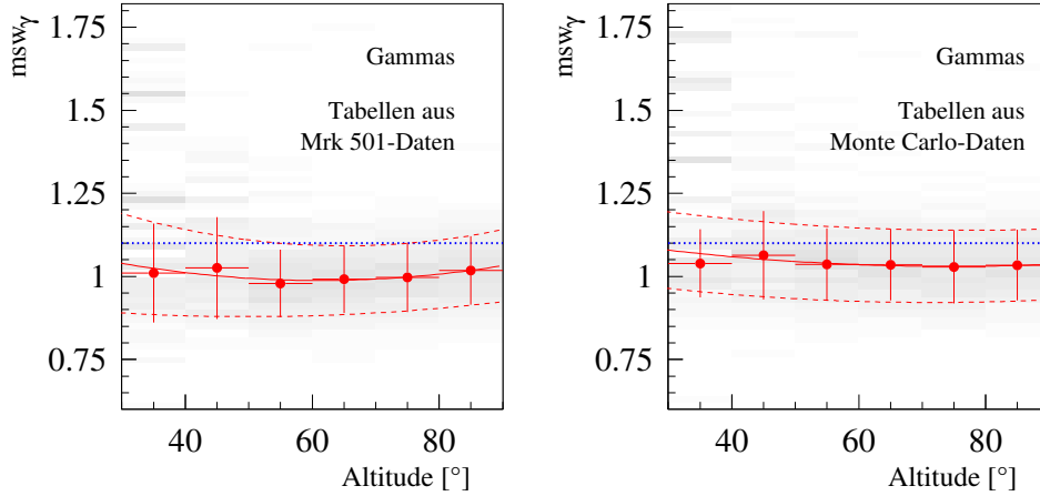
Abbildung 7.4: Vergleich der \gamma -mean scaled width-Verteilungen des Krebsnebel Datensatzes unter Anwendung der aus den Mrk 501-Daten gewonnenen \gamma -Erwartungswerte (links) und bei Verwendung der Monte Carlo-Tabellen (rechts). Zur Bestimmung der durchgezogenen und gestrichelten Kurven siehe die Beschreibung zu Abb. 7.2. Die gepunktete Linie zeigt die Position des msw < 1.1 -Schnitts an. Generell ist eine gute Übereinstimmung der beiden Parametrisierungen zu erkennen. Die Verteilung rechts weicht jedoch um 3-4% von der Erwartung ab, daß die mean scaled width bei 1 zentriert sein sollte.
