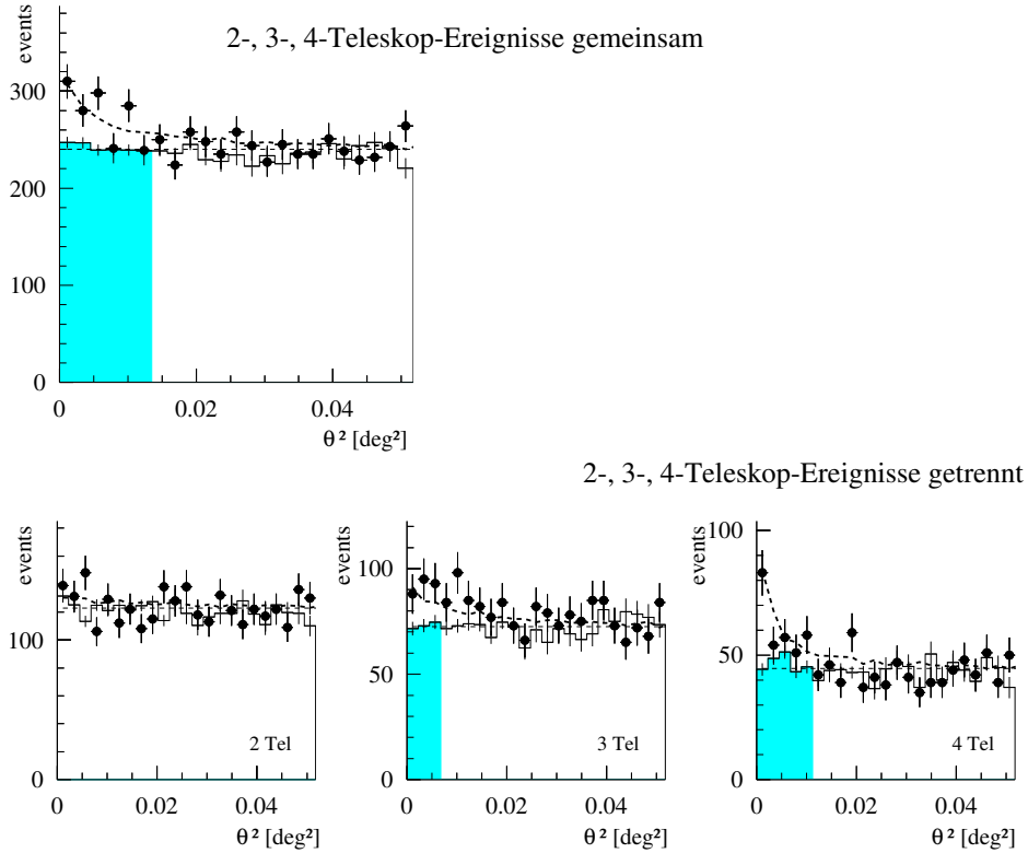
Abbildung 9.11: Winkelverteilung des Cas A-Datensatzes. Oben sind alle Ereignisse in einem Histogramm zusammengefaßt (normale \theta^2 -Darstellung), unten sind die Ereignisse nach der Zahl der effektiv am Ereignis beteiligten Teleskope getrennt dargestellt. Für alle Daten gilt ein mean scaled width -Schnitt von 0.5 < msw < 1.1 . Die gefüllten Punkte geben die Ereigniszahlen bezüglich der Cas A-Position an. Die mit durchgezogenen Linien dargestellten Histogramme sind die Untergrundverteilungen. Im Bereich der optimalen Winkelschnitte sind die Untergrundhistogramme grauschattiert dargestellt. Die fettgestrichelten Linien sind die Krebsnebel- \gamma -Ereignisverteilungen in dem zu den Cas A-Daten korrespondierenden Zenitwinkelbereich, normiert auf die ermittelte Cas A-Flußstärke; sie wurden zu den durch die feingestrichelten Linien dargestellten Untergrundniveaus hinzuaddiert, welche aus den jeweils ersten 10 Bins der Untergrundverteilungen gewonnen werden.
