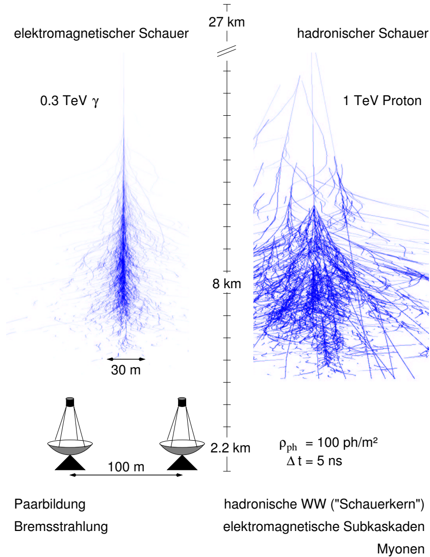
Abbildung 2.1: Eigenschaften ausgedehnter Luftschauer, die von Primärteilchen im TeV-Energiebereich ausgelöst werden. Die Schauerbilder spiegeln die Cherenkov-Emissionsdichte wieder. Beide dargestellten Schauer erzeugen in der Analyse ein Bild mit etwa derselben Amplitude; zu höheren Energien wird der Energieunterschied von hadronischen und elektromagnetischen Schauern mit gleicher Bildamplitude deutlich geringer (ca. 20% bei 10 TeV). Primäre \gamma 's (oder Elektronen) induzieren praktisch reine elektromagnetische Schauer aus Elektronen und \gamma 's; der Transversalimpulsübertrag der Wechselwirkungen ist gering, es entwickeln sich kompakte Schauer. Primäre Hadronen induzieren aufgrund des höheren Transversalimpulses der hadronischen Wechselwirkung deutlich diffusere Bilder; dieser Unterschied erlaubt die (statistische) Unterscheidung von primären \gamma 's und Hadronen aufgrund von Schauerformparametern.
