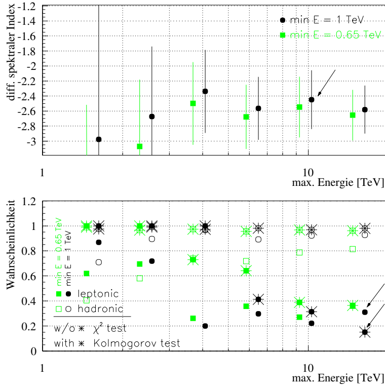
Abbildung 10.11: Ergebnisse der a posteriori durchgeführten Tests zur Beschreibung des Cas A- \gamma -Spektrums unter Anwendung verschiedener Energiebereiche. Oben sind die Ergebnisse der Fits an ein Potenzgesetz gezeigt, unten die Ergebnisse der \chi^2 - und der Kolmogorov-Tests. Für das untere Ende der Energieskala wurde 1 TeV (dunkle Symbole) und 0.65 TeV (graue Symbole) gewählt. Das obere Ende des Energiebereiches wird durch die Abszisse angegeben. Die Ergebnisse für die in der Analyse a priori ausgewählten Energiebereiche sind durch Pfeile markiert.
