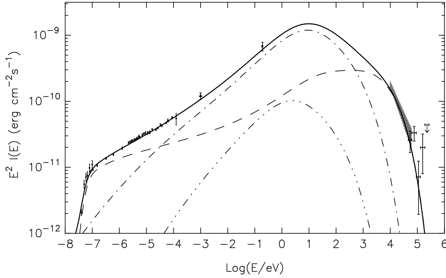
Abbildung 11.2: Breitband-Synchrotronspektrum von Cassiopeia A. Die Daten reichen vom Radio- bis in den Röntgenspektralbereich. Die Modellkurve (durchgezogene Linie) wird im Rahmen des diskutierten Teilchentransportmodells erzeugt und setzt sich aus Beiträgen von drei Emissionszonen zusammen, die durch ihre Magnetfelder charakterisiert werden: B_1 = 1.6 mG (gestrichelte Kurve), B_2 = 0.4 mG (strichpunktiierte Linie) und B_3 = 0.1 mG (Dreipunkt-Strich-Linie). Zu Details siehe Text. Aus [AATV00].
