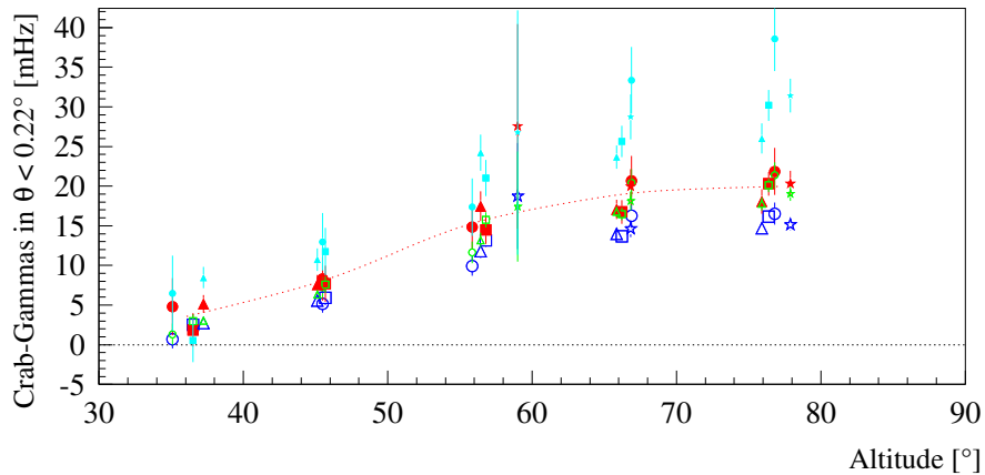
Abbildung 5.3: Krebsnebel- \gamma -Raten, aufgeteilt in dieselben Zenitwinkelbereiche und Zeitabschnitte wie oben. Die Symboldefinition stimmt ebenfalls überein, jedoch wurden die Raten ohne Softwareschwelle mit Schauerformschnitt der Übersichtlichkeit halber weggelassen. Auch die \gamma -Rate nach Anwendung der Softwareschwelle ist im wesentlichen zeitlich konstant; es gibt jedoch noch leichte Schwankungen (bis 10%), die etwas über den statistischen Fehler hinausreichen.
