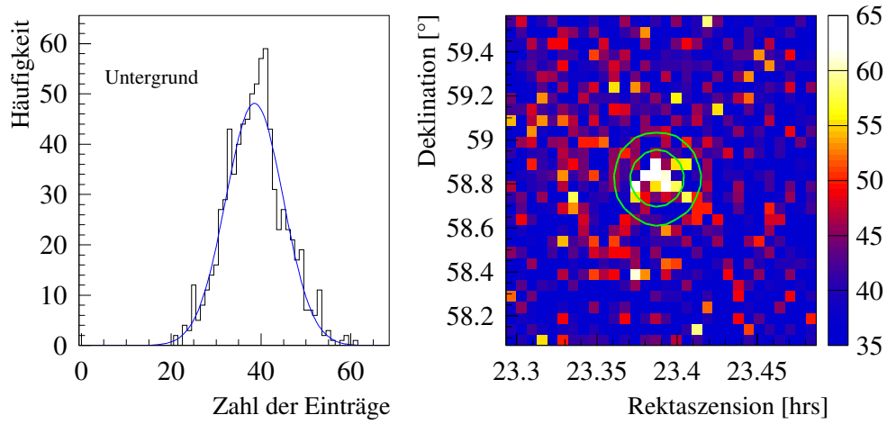
Abbildung 9.1: Richtungsrekonstruktion am Beispiel des vollen Cas A-Datensatzes. Links: Histogrammierte Untergrundverteilung; der Mittelwert der gefitteten Gaußkurve (bzw. der Erwartungswert einer gefitteten Poissonverteilung im Falle kleiner Statistik) wird als Untergrunderwartung bei der Bestimmung der Quellposition verwendet. Rechts: Zweidimensionale Ereignisverteilung in Himmelskoordinaten in einem 0^{\circ}05 \times 0^{\circ}05 -Histogramm. Das Bild wurde etwas „geschönt“, indem das Minimum der Farbskala von 21 auf 35 erhöht und das Maximum von 68 auf 65 gesenkt wurde. Die Kreise zeigen die 68%- und 95%-Radien der gefitteten 2-dimensionalen Gaußfunktion an, aus der der Schwerpunkt der TeV-Emission bestimmt wird.
