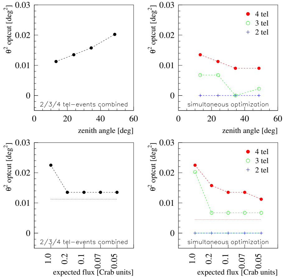
Abbildung 9.12: Winkelschnittoptimierung mit Hilfe des kombinierten Krebsnebel- und Mrk 501-Datensatzes. Oben links: optimaler Winkelschnitt der normalen Winkelverteilung, in der alle Ereignisse gemeinsam ausgewertet werden, für einen erwarteten Fluß von 5% des Krebsnebelflusses, als Funktion des Zenitwinkels. Oben rechts: Optimale Winkelschnitte für dieselbe Flußerwartung, wenn die Ereignisse getrennt nach der Zahl der effektiv am Ereignis beteiligten Teleskope ausgewertet werden. Unten links: optimaler Winkelschnitt der alle Ereignisse umfassenden Winkelverteilung für den Zenitwinkelbereich zwischen 20^\circ und 30^\circ , als Funktion des erwarteten Flußniveaus. Die gepunktete Linie gibt die Position des Q -Faktor-optimierten Winkelschnitts an. Unten rechts: Dieselbe Auftragsung für die nach der Zahl der Teleskope getrennte Auswertung der Winkelverteilung. Die Q -Faktor-Optimierung liefert in diesem Fall einen Winkelschnitt von \theta_{\text{opt},4\text{tel}} = 0.0045^\circ für 4-Teleskop-Ereignisse, und die völlige Zurückweisung der weiteren, mit weniger Teleskopen erfaßten Ereignisse.
