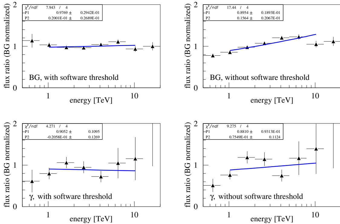
Abbildung 10.4: Derselbe Vergleich wie in Abb. 10.3, mit den Daten unter Zenitwinkeln 25^\circ - 40^\circ ( \gamma -Spektren: msw < 1.2 ). Der getestete Energiebereich liegt bei 1-10 TeV, der auch bei der Bestimmung des Cas A-Spektrums verwendet wird.
