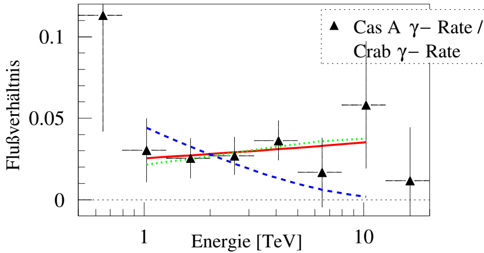
Abbildung 10.8: Vergleich der \gamma -Rohspektren des Cas A- und des Krebsnebel Datensatzes (Zenitwinkel 25^\circ - 40^\circ ). Auf die Daten wurden harte Schnitte angewendet ( 0.5 < m_{sw} < 1.1 , \theta^2 < 0.0135^\circ^2 ). Die Zahlen der Krebsnebel- \gamma -Ereignisse wurden entsprechend der unterschiedlichen Beobachtungszeiten der beiden Datensätze hochskaliert. Das Bild zeigt das in Gl. 10.5 beschriebene Spektrum, in dem die \gamma -Ereignisse des Cas A- und des Krebsnebel Datensatzes binweise dividiert werden. Die Fehler werden mittels Gaußscher Fehlerfortpflanzung berechnet. Unter der Annahme, daß beide Spektren aus Quellspektren stammen, die einem Potenzgesetz folgen, sollte dieses Verhältnis wiederum einem Potenzgesetz \propto E^{\Delta\alpha} folgen; die durchgezogene Linie zeigt den entsprechenden Fit für den Energiebereich zwischen 1 und 10 TeV. Außerdem sind Anpassungen der hadronischen (gepunktete Linie) und der leptonischen (gestrichelte Linie) Modellspektren gezeigt, die in Abschnitt 10.7 diskutiert werden; in diesem Fall liegt der für die Anpassung verwendete Energiebereich bei 1 bis 20 TeV.
