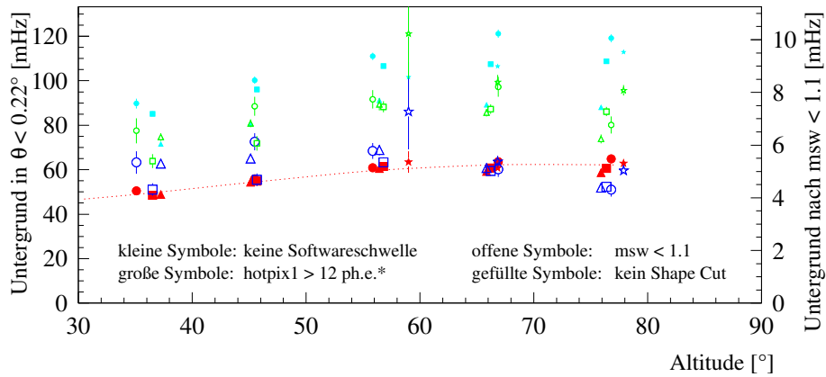
Abbildung 5.2: Untergrundraten in den Krebsnebeln, die in verschiedene Zenitwinkelbereiche und Zeitabschnitte aufgeteilt wurden; die letzteren sind in Tabelle 5.2 definiert. Für die Raten ohne Schauerformschnitt gilt die linke vertikale Achse, für die Raten mit Schauerformschnitt ( mean scaled width < 1.1) die rechte Achse. Die großen gefüllten Symbole zeigen die Raten nach Softwareschwelle an; diese sind erwartungsgemäß innerhalb weniger Prozent zeitlich konstant. Die gepunkteten Linien sind in dieser und in der unteren Abbildung manuell hineingemalt worden, um das Auge entlang der Raten nach Softwareschwelle (ohne Schauerformschnitt) zu führen.
