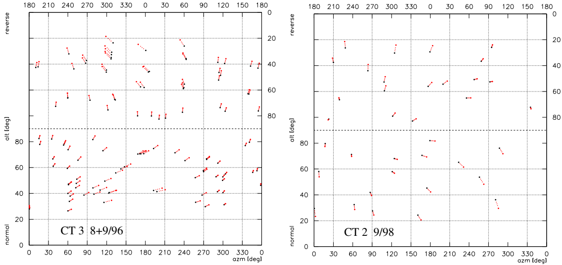
Abbildung 4.7: Ergebnisse zweier Ausrichtungskalibrationen. Der Ursprung der „Pfeile“ ist an der jeweiligen Position des Teleskops während des Point Runs in erdfesten Azimutal-Koordinaten gezeichnet. Die Richtungen und Längen geben die Verschiebungsvektoren in der Kameraebene wieder; sie sind um ca. einen Faktor 50 vergrößert, um in dieser Darstellung sichtbar zu werden.
