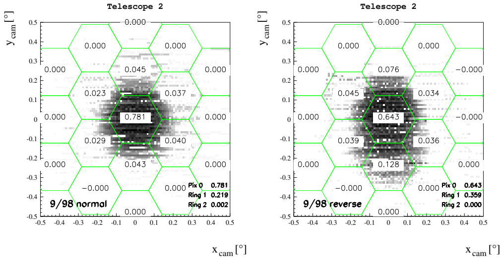
Abbildung 4.12: Die Punktantwort von CT 2 direkt nach seinem Einschluß in das Teleskopsystem, getrennt nach normal und reverse mode . Die Spiegeljustierung findet bei horizontaler Ausrichtung des Teleskops im normal mode statt, in diesem Modus scheint die Punktantwort noch akzeptabel. Im reverse mode dagegen ist eine deutliche Störung zu erkennen.
