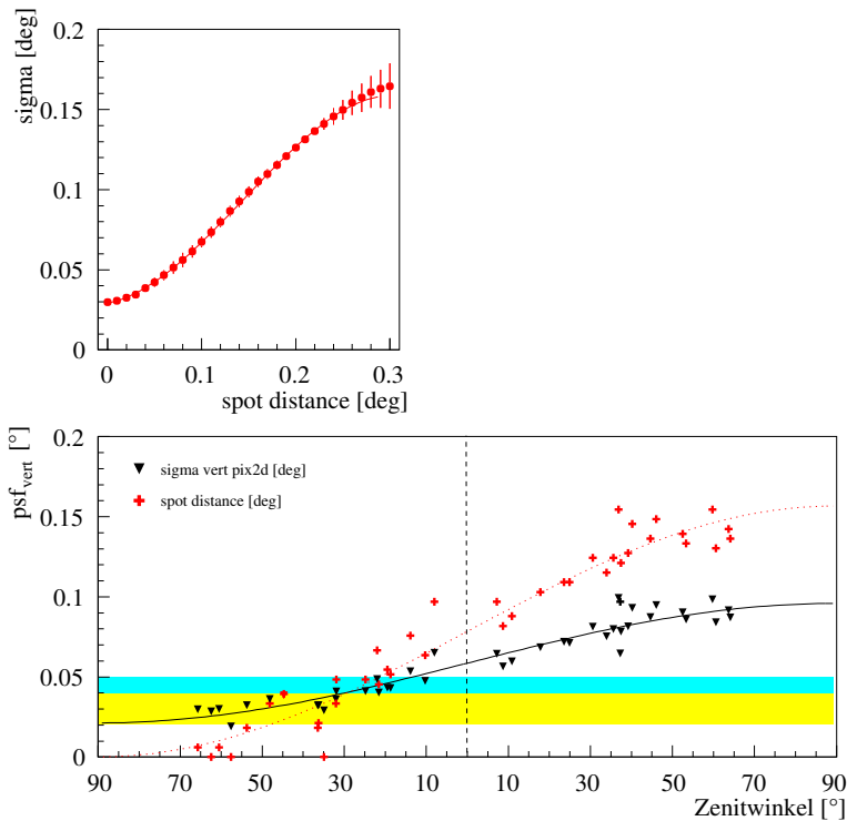
Abbildung 4.14: Einfache Simulation des Reflektorverhaltens von CT2. Oben: Zusammenhang zwischen der Entfernung zweier Lichtflecke (Intensitätsverhältnis 2:1), aus denen sich die PSF zusammensetzt, und der gemessenen Breite der PSF . Unten: Unter der Annahme, daß sich die Entfernung der Lichtflecke wie ein typischer Durchbiegungseffekt verhält, gibt die Simulation genau die gemessenen Breiten wieder.
