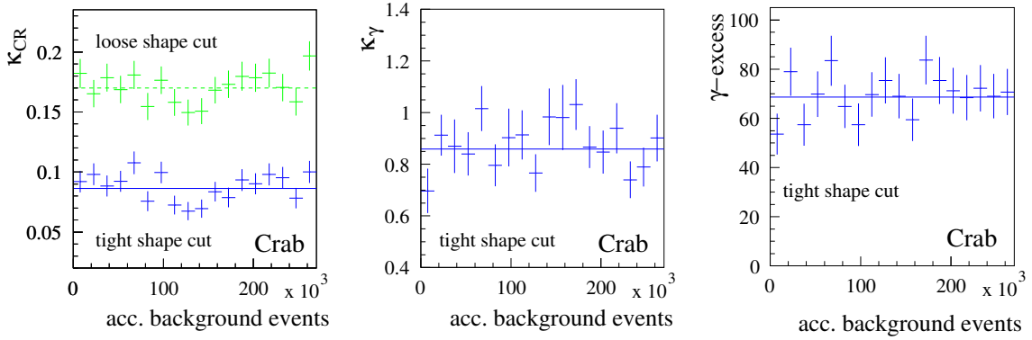
Abbildung 7.10: Dieselben Daten wie in Abb. 7.9, allerdings nach Anwendung der Software-schwelle zum spektralen Akzeptanzausgleich.
