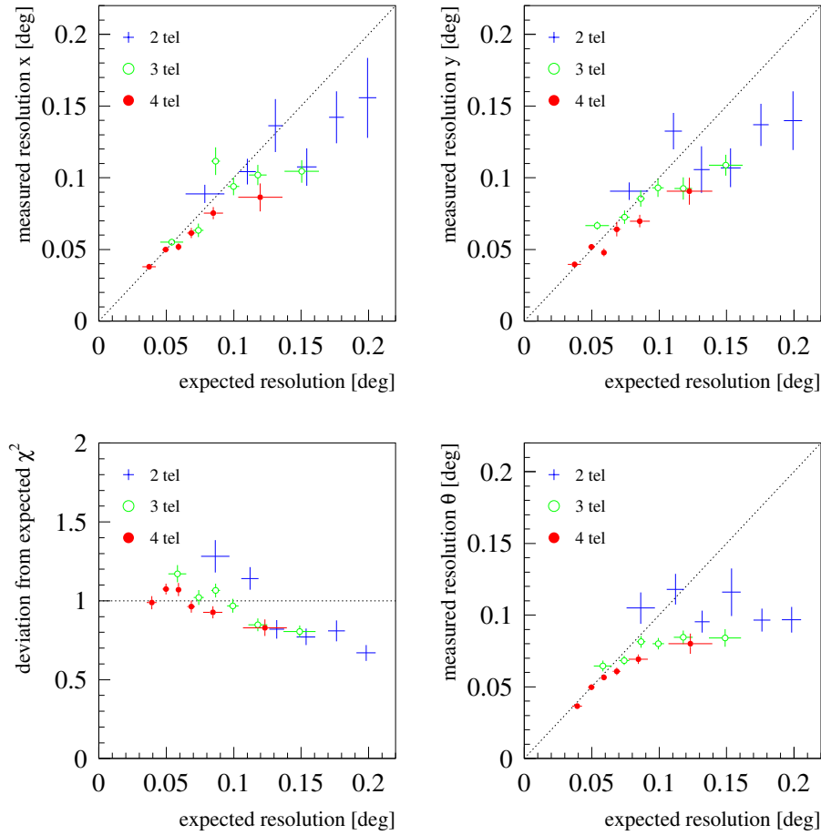
Abbildung 9.9: Ergebnisse der Tests über die Richtungsfehlervorhersage für die Daten bei kleinen Zenitwinkeln (bis 20^\circ ). Oben: Projektionen in x und y . Unten links: \chi^2 -Test. Innerhalb von 15% stimmen die Vorhersage und der rekonstruierte Richtungsfehler überein. Unten rechts: Bis zu einem Richtungsfehler von 0^\circ.1 gibt die Annahme einer (nahezu) sphärischen Kovarianzmatrix gute Vorhersagen für die gemessene Breite der \theta^2 -Verteilung. Wie erwartet, lassen sich 2-Teleskop-Ereignisse nicht gut auf diese Weise charakterisieren.
