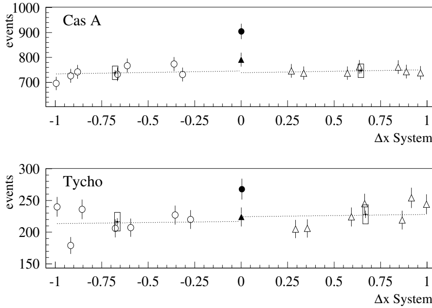
Abbildung 8.6: Ereigniszahlen in den Kontrollregionen des Cas A- und des Tycho-Datensatzes nach Anwendung harter Schnitte ( msw < 1.1, \theta^2 < 0.0135^\circ^2 ), aufgetragen als Funktion der x_{\text{system}} -Koordinate.
