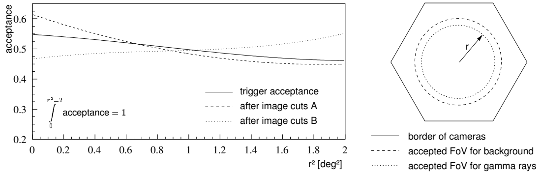
Abbildung 5.6: Radiale Untergrundakzeptanz im Gesichtsfeld des HEGRA-Systems. Gezeigt ist eine Parametrisierung, die mit den Daten des ersten Scans der Galaktischen Ebene gewonnen wurde, für alle Untergrundereignisse ( trigger acceptance ) und zwei Schauerformschnitte (den sogenannten MHD-Cut und den probability cut , siehe Kap. 7.7). Man erkennt, daß die Akzeptanz deutlich von den verwendeten Schauerformschnitten abhängt.
