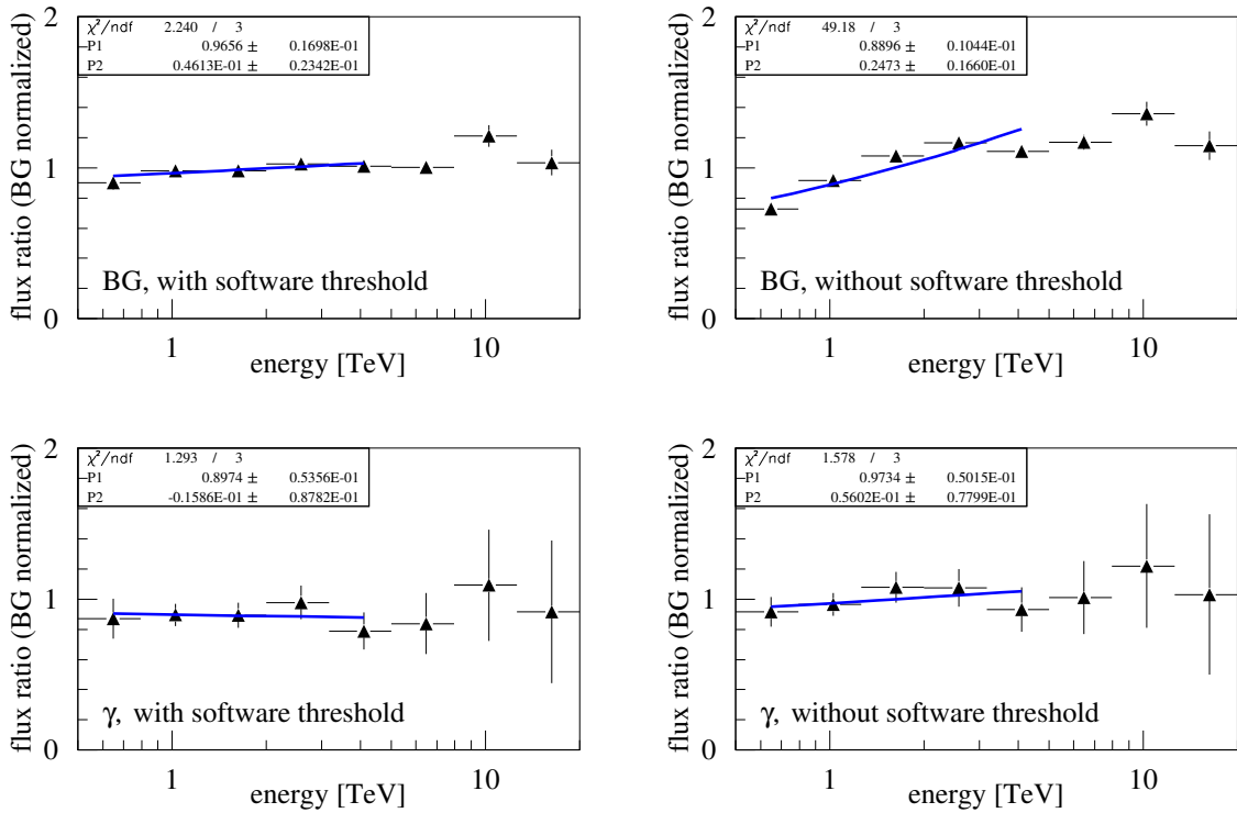
Abbildung 10.3: Vergleich der Untergrundspektren (oben) und der \gamma -Spektren (unten) zweier jahresweise zusammengefaßten Krebsnebel Datensätze (Winter 98/99 im Vergleich zum Winter 97/98, Zenitwinkel 0^\circ - 25^\circ ). Untergrundspektren: \theta^2 < 0.0225^\circ^2 , kein Schauerformschnitt. \gamma -Spektren: \theta^2 < 0.0135^\circ^2 , m_{sw} < 1.1 ). Gezeigt ist jeweils das Verhältnis zweier Rohspektren, die Datensätze wurden entsprechend dem Verhältnis der Gesamtzahl der Untergrundereignisse normiert. An die Daten wurde jeweils ein Potenzgesetz angepaßt; bei Übereinstimmung der spektralen Akzeptanzen sollte der angepaßte Exponent klein sein, der Vergleich sollte näherungsweise eine Waagerechte ergeben. Der getestete Energiebereich liegt zwischen 500 GeV und 5 TeV. Links ist jeweils der Vergleich der Spektren unter Anwendung der Softwareschwelle gezeigt. Man erkennt im Rahmen des statistischen Fehlers die erwartete gute Übereinstimmung der spektralen Akzeptanz, sowohl für Hadronen wie auch für \gamma -Ereignisse. Rechts ist derselbe Vergleich ohne Einsatz der Softwareschwelle gezeigt.
