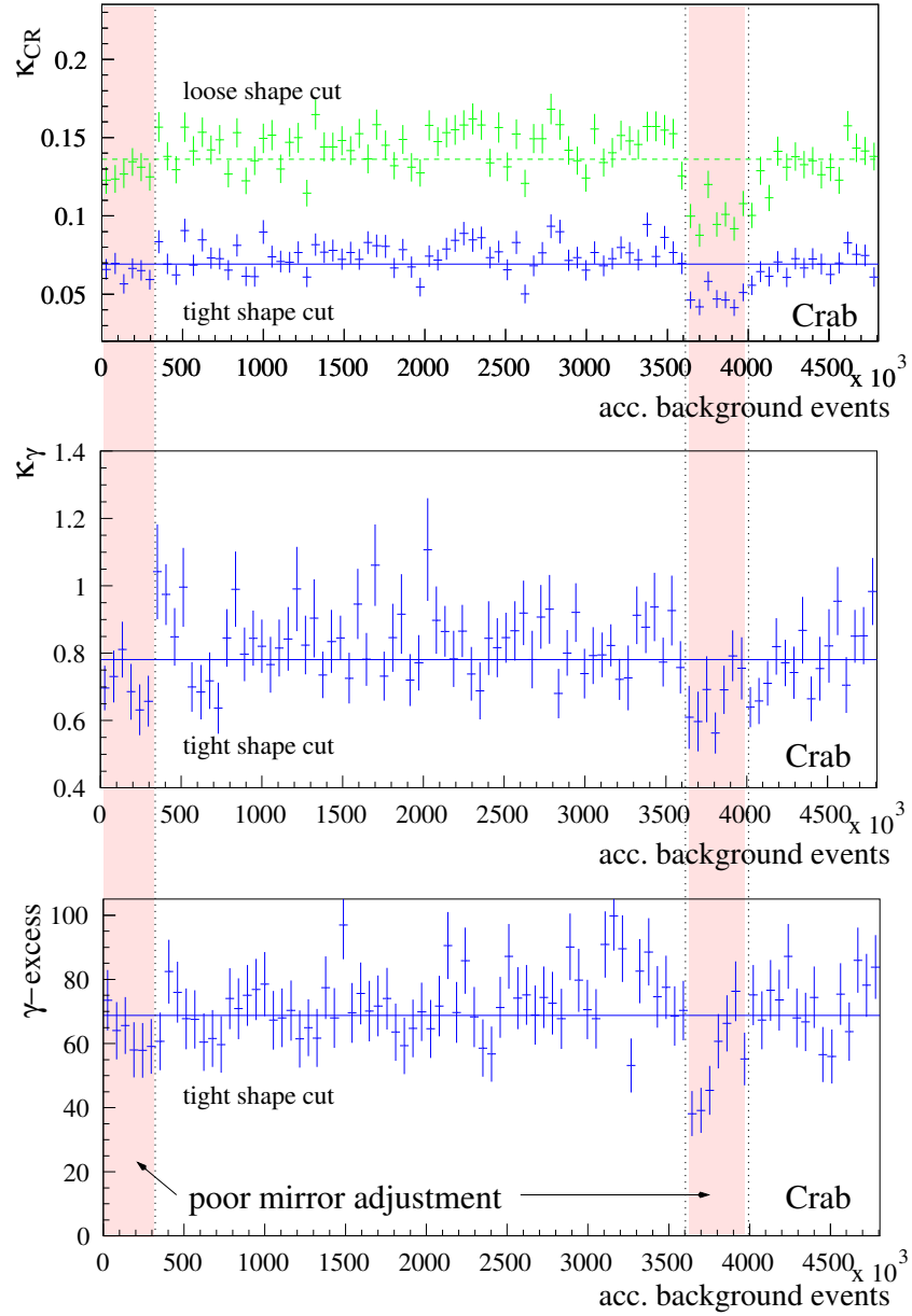
Abbildung 7.6: Schnitteffizienzen und \gamma -Rate des Krebsnebel Datensatzes als Funktion der akkumulierten Ereignisse für Daten zwischen 0^\circ und 25^\circ Zenitwinkel. Ein Bin entspricht ca. einer Stunde Datennahme unter optimalen Detektorbedingungen (15 Hz Datenrate). Oben: Untergrundunterdrückung für den lockeren ( msw < 1.2 ) und den harten ( msw < 1.1 ) Schauerformschnitt. Mitte: \gamma -Effizienz des harten Schnitts. Diese Werte werden aus einem Vergleich der untergrundsubtrahierten Ereignisse mit Ereignissen gewonnen, auf die nur ein Schnitt von msw < 1.4 angewandt wurde; dieser verwirft de facto keine \gamma -Ereignisse. Unten: Crab- \gamma -Ereignisse nach Anwendung des harten Schnitts. Für die Daten wurde ein Winkelschnitt von \theta^2 < 0.0225^\circ^2 verwendet; der Untergrund wird aus dem 7-Kontrollregionen-Aufbau gewonnen (Kap. 8.3.3).
