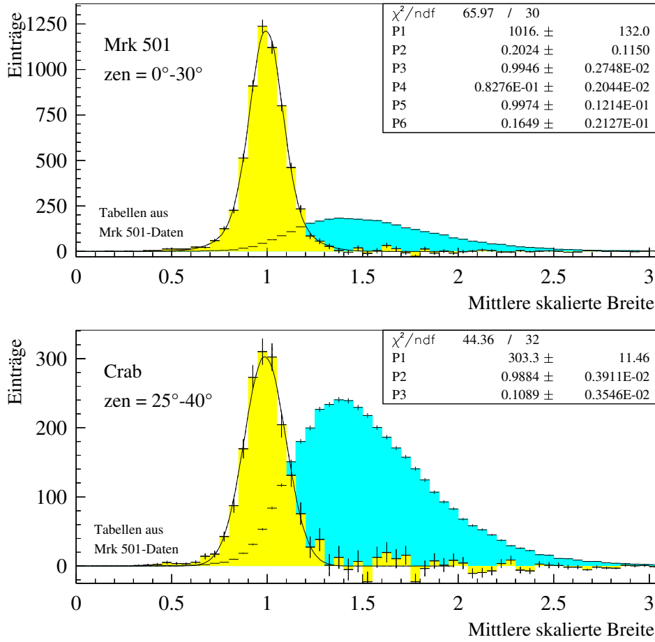
Abbildung 7.3: Mittlere skalierte Breite der \gamma -Ereignisse (hellschattierte Histogramme) und der Untergrundereignisse (dunkelschattierte Histogramme), am Beispiel der Mrk 501-Daten bei kleinen Zenitwinkeln (oben) und der Krebsnebel Daten bei mittleren Zenitwinkeln (unten). Die \gamma - m_{sw} -Verteilung lässt sich bei ausreichender Statistik durch eine Doppelgaußfunktion, bei geringerer Statistik annähernd durch eine einfache Gaußfunktion parametrisieren.
