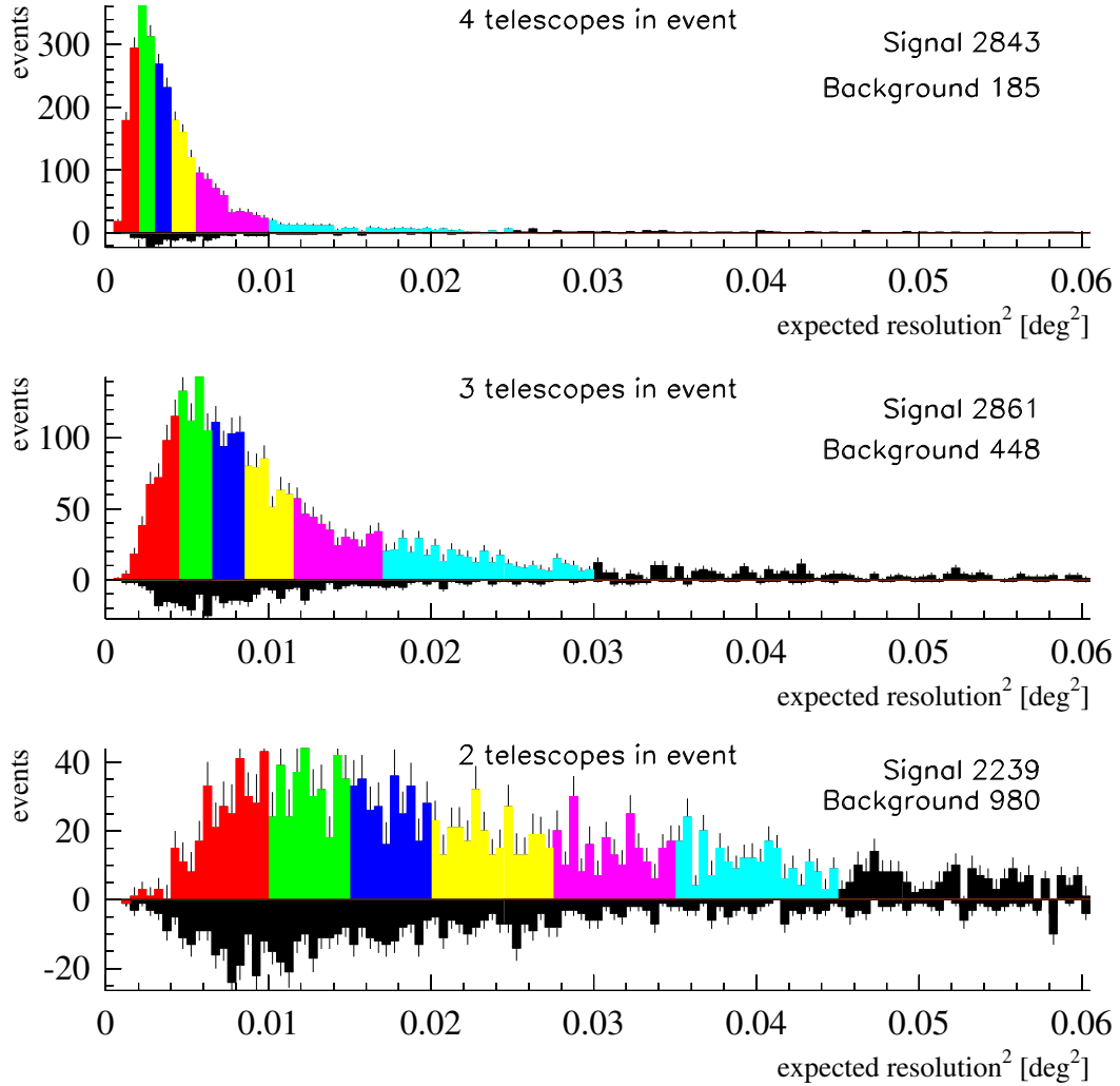
Abbildung 9.7: Verteilung der Erwartungswerte für den Richtungsfehler \langle x^2 \rangle . Die Daten stammen von echten \gamma -Ereignissen von Mrk 501 und dem Krebsnebel, die unter einem Zenitwinkel von weniger als 20^\circ genommen wurden. Ein Winkelschnitt von \theta^2 < 0.014^\circ und ein Schauerformschnitt von msw < 1.1 wurden verwendet, um \gamma 's zu selektieren. Die Ereignisse wurden nach der Zahl der effektiv am Ereignis beteiligten Teleskope aufgeteilt. Die schwarzen Histogramme zeigen die zur Signalregion gehörige Untergrunderwartung (multipliziert mit -1). Man erkennt erwartungsgemäß, dass die Richtungsauflösung mit der Zahl der an der Rekonstruktion beteiligten Teleskope ansteigt. Die unterschiedlichen Graustufen der Signalhistogramme markieren die Ereignisklassen, die in den nachfolgenden Abbildungen getrennt getestet wurden.
