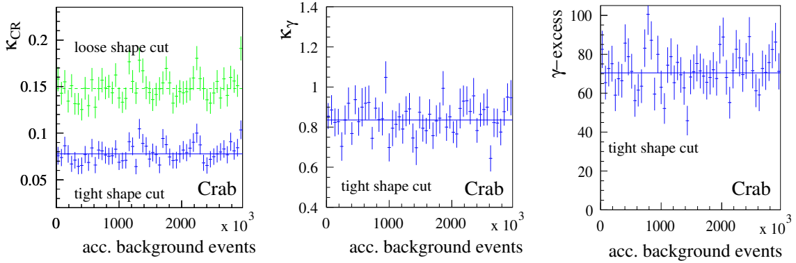
Abbildung 7.8: Dieselben Daten wie in Abb. 7.7, allerdings nach Anwendung der Software-schwelle zum spektralen Akzeptanzausgleich.
