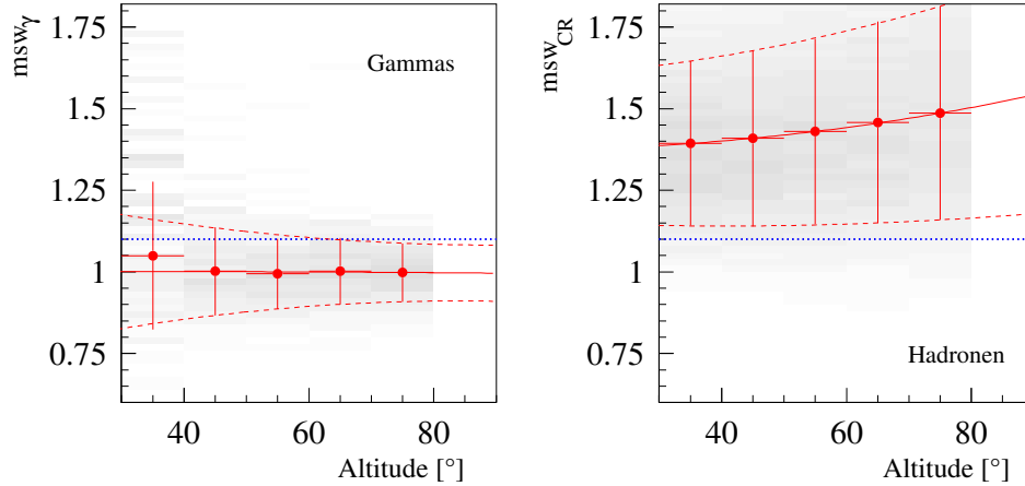
Abbildung 7.2: Mittlere skalierte Breite der Mrk 501-Daten, oben ohne, unten mit Zenitwinkelskalierung, links für \gamma 's, rechts für Untergrundereignisse. Die Daten sind in 10^\circ breite Zenitwinkelabschnitte aufgeteilt. Die Punkte geben jeweils den Schwerpunkt, die Fehlerbalken die Breite einer an die Verteilung angepaßten einfachen Gaußfunktion an. Die durchgezogene Kurve zeigt jeweils das Ergebnis einer Anpassung eines Polynoms zweiten Grades an die Schwerpunkte an. Die Breite der an die mittlere skalierte Breite angepaßten Gaußfunktion wird ebenfalls durch eine Anpassung eines Polynoms zweiten Grades beschrieben; das Ergebnis wird zu der durchgezogenen Kurve addiert bzw. abgezogen und als gestrichelte Linien in die Abbildungen eingezeichnet, um das Auge zu leiten. Nach Anwendung der Zenitwinkelskalierung ist die mean scaled width -Verteilung der \gamma 's erwartungsgemäß für alle Zenitwinkel bei 1 zentriert. Die Untergrundverteilung rückt mit zunehmendem Zenitwinkel näher an die \gamma -Verteilung heran.
