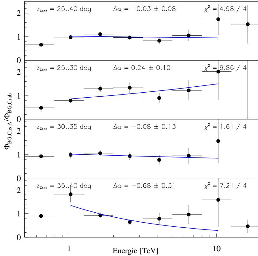
Abbildung 10.6: Vergleich der Untergrundspektren des Cas A- und des Krebsnebel Datensatzes; es wurde ein lockerer Winkelschnitt, aber derselbe Schauerformschnitt wie bei der Bestimmung der \gamma -Spektren gewählt. Die Untergrundspektren sind ein gutes Maß auch für die Übereinstimmung der spektralen \gamma -Akzeptanz. In allen vier Spektren wird der volle Cas A-Datensatz verglichen: oben mit dem vollen Krebsnebel-Referenzdatensatz zwischen 25^\circ und 40^\circ Zenitwinkel und in den weiteren Abschnitten jeweils mit Unterbereichen von 5^\circ Breite. Man erkennt erwartungsgemäß die beste Übereinstimmung im Falle der 30^\circ - 35^\circ -Krebsnebel Daten. Ähnlich gute Übereinstimmung wird aber auch bei dem vollen 25^\circ - 40^\circ -Abschnitt erreicht, allerdings unter Auslassung des niedrigsten Energiebins (500 GeV-1 TeV). Aus diesem Grund wurde in der Cas A-Spektrumsanalyse a priori dieses Energiebin ausgelassen.
