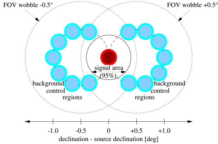
Abbildung 8.3: Aufbau der Kontrollregionen für die im Wobble Mode genommenen Daten, der in dieser Arbeit zur Bestimmung des erwarteten Untergrundes in der Signalregion genutzt wird. Der Rand des effektiven Gesichtsfeldes wird durch die gepunkteten Kreise gezeigt; die Gesichtsfelder sind um \pm 0.5^\circ in Richtung der Deklination von der Quellposition versetzt. Auf einem Kreis mit dem Radius 0.5^\circ um den Ursprung des Gesichtsfeldes befinden sich sowohl die Signalregion wie auch alle Untergrundkontrollregionen; der Kreis wird durch eine gestrichelte Linie ansatzweise angedeutet. Auf diese Weise wird sichergestellt, daß für alle Winkelschnitte bis \theta = 0.15^\circ die radiale Akzeptanz für Signal- und Untergrundmessungen identisch ist. Die Untergrundregion ist innerhalb dieses Bereichs immer siebenmal größer als die Signalregion. Die dunkelschattierten Bereiche der Kontrollregionen entsprechen dem für die Quellsuche optimalen Winkelschnitt von \theta_{\text{opt,int}}^2 = 0.0135^\circ{}^2 (siehe Kap. 9.3.2).
