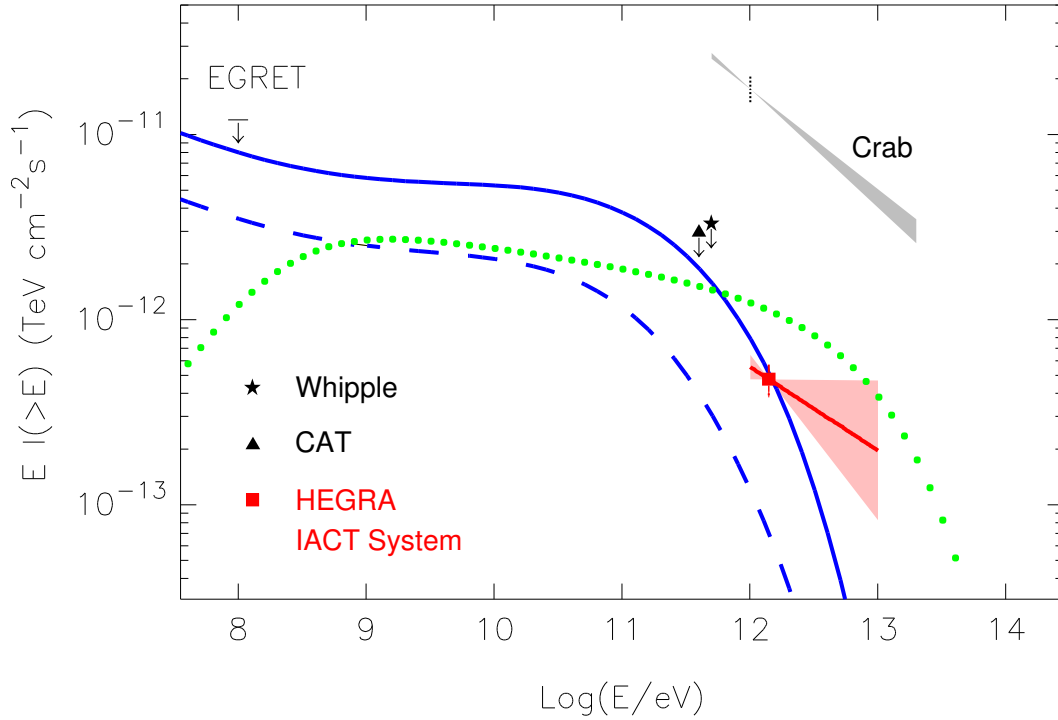
Abbildung 11.4: Der gemessene integrale Fluß von Cassiopeia A (gefülltes Quadrat) zusammen mit dem 1\sigma -Fehlerbalken des aus dem differentiellen spektralen Index berechneten integralen Spektrums zwischen 1 und 10 TeV (grauschattiertes Feld); das Spektrum gilt unter der Annahme eines Potenzgesetzes. Zum Vergleich ist das Krebsnebelspektrum zwischen 1 und 20 TeV eingetragen. Außerdem sind die oberen Flußgrenzen für Cas A von EGRET, Whipple und CAT eingezeichnet. Die Beobachtungen werden mit Modellvorhersagen verglichen. Die gepunktete Linie gibt das aus hadronischen Modellen hergeleitete Spektrum wieder; die Absolutnormierung der Vorhersage ist allerdings in gewissen Grenzen variabel. Die durchgezogene Linie und die gestrichelte Linie sind die im Rahmen der leptonischen Modelle vorhergesagten IC- plus Bremsstrahlungsflüsse für zwei verschiedene Parameterwerte ( B_1 = 1 mG bzw. B_1 = 1.6 mG).
