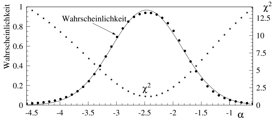
Abbildung 10.9: Reduziertes \chi^2 und die daraus abgeleitete Wahrscheinlichkeit für verschiedene spektrale Indizes, wenn das Cas A- \gamma -Spektrums mit einem Potenzgesetz zwischen 1 und 10 TeV beschrieben wird. Der Verlauf der Wahrscheinlichkeit wird durch eine Gaußfunktion beschrieben (durchgezogene Kurve).
