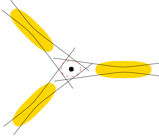
Abbildung 9.6: Skizze zur Erläuterung der Fehlerbestimmung bei der stereoskopischen Rekonstruktion. Die durch die lange Halbachse der Ellipse rekonstruierte Schauerrichtung hat einen Winkelfehler; zusätzlich wird der Fehler der Schwerpunktsbestimmung senkrecht zu der (rekonstruierten) Schauerachse berücksichtigt. Als rekonstruierte Schauerrichtung wird der Punkt gewählt, der den Abstand zu den rekonstruierten Schauerachsen minimiert; als Abstand wird die Summe der mit den entsprechenden Fehlern gewichteten Abstände zu den Schauerachsen verwendet. Gleichzeitig erhält man auf diese Weise eine Fehler-Kovarianzmatrix. Aus [HJK + 99].
