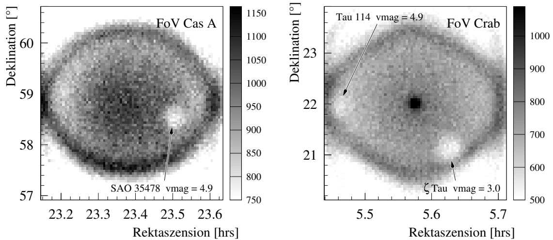
Abbildung 8.7: Gesichtsfelder des Cas A-Datensatzes (links) und des Krebsnebel-Datensatzes (rechts) in Himmelskoordinaten. Gezeigt sind alle Ereignisse ohne Schauerformschnitt. Sterne im Gesichtsfeld führen zu einem Defizit in der Untergrundverteilung innerhalb des FOV. Darüberhinaus ist die Abnahme der rekonstruierten Ereignisse mit Abstand zur Bildfeldmitte zu erkennen. An den Rändern der Gesichtsfelder (die im Wobble Mode abwechselnd um +0.5^\circ und -0.5^\circ gegen die Deklination der Quelle verschoben sind) ist eine Häufung von rekonstruierten Ereignissen zu sehen, die durch abgeschnittene Schauerbilder an den jeweiligen Kamerarändern verursacht wird.
