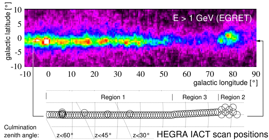
Abbildung 5.4: Übersicht über die Positionen, die im ersten Scan der Galaktischen Ebene mit dem HEGRA-System abgesucht wurden. Das Ziel war eine Suche nach neuen TeV- \gamma -Punktquellen mit einer Empfindlichkeit von deutlich weniger als einem Crab.
