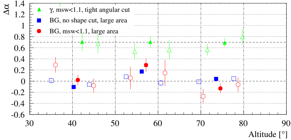
Abbildung 10.2: Ergebnisse der Vergleiche der Rohspektren von Mrk 501 und dem Krebsnebel als Funktion des untersuchten Zenitwinkelbereichs. Die gefüllten Symbole entsprechen den Ergebnissen der Zenitwinkelabschnitte 0^\circ - 25^\circ , 25^\circ - 40^\circ und 40^\circ - 60^\circ . Außerdem wurden diese Zenitwinkelabschnitte noch einmal halbiert, die Ergebnisse sind als offene Symbole dargestellt. Die \gamma -Erwartungswerte (Dreiecke) stimmen im Rahmen der statistischen Fehler mit dem erwarteten Wert von \Delta\alpha \approx 0.7 überein. Zu weiteren Details siehe Text.
