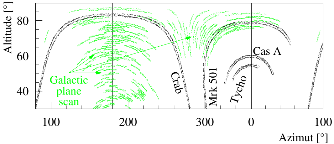
Abbildung 5.1: Übersicht über die Teleskopausrichtungen, unter denen die in dieser Arbeit untersuchten Daten aufgezeichnet wurden. Die Doppellinien bei den Punktquellen rühren von dem Wobble -Beobachtungsmodus her (alternierender Versatz um \Delta dec = \pm 0.5^\circ zur Quellposition). Für den überwiegenden Teil der Analyse ist nur der Zenitwinkel der Beobachtungen relevant; mit ihm ändern sich Energieschwelle und -eichung, Ereignisrate und die erwarteten Schauerformparameter. Nur für genaue Untersuchungen der Homogenität des Gesichtsfeldes ist die volle Ausrichtung von Bedeutung (siehe Kap. 8.3.1). Der Azimut-Bereich der Abbildung von ganz links bis zur Mitte ( 80^\circ bis 280^\circ ) wird im „normalen“ Modus, der übrige Bereich im „reversen“ Modus beobachtet. Auf diese Weise wird gewährleistet, daß für jede Quelle eine durchgängige Beobachtung ohne Beschränkung durch die toten Bereiche der Teleskopausrichtung möglich ist (siehe Kap. 4.3.2).
