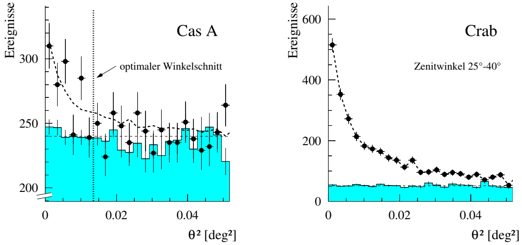
Abbildung 6.1: Verteilung der Ereignisse als Funktion des Quadrats des Abstands zur Quell- bzw. zu den Kontrollpositionen im Gesichtsfeld (sogenannte \theta^2 -Auftragung). Links ist das Ergebnis aus den Cas A-Daten gezeigt, rechts der Krebsnebel-Referenzdatensatz, der unter ähnlichen Zenitwinkeln wie der Cas A-Datensatz aufgezeichnet wurde. Alle Daten wurden nach einem Schauerformschnitt von 0.5 < msw < 1.1 gewonnen. Die gefüllten Punkte sind die Ereigniszahlen bezüglich der jeweiligen Quellposition, das grauschattierte Histogramm zeigt die auf die Signalregion normierte Summe der Untergrundmessungen. Die vertikale gepunktete Linie gibt die Position des optimalen Winkelschnitts an. Die gestrichelte Linie in der Cas A-Verteilung (links) zeigt die Krebsnebel- \gamma -Ereignisverteilung, die aus dem rechten Histogramm gewonnen wurde; die Daten wurden auf die ermittelte Cas A-Flußstärke (3% Crab) normiert und zu einer flachen Untergrundverteilung addiert.
