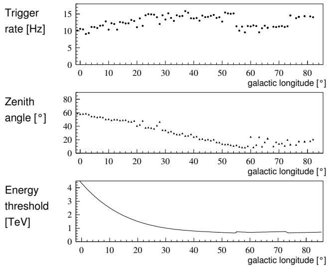
Abbildung 5.5: Einige Charakteristika zum ersten Scan der Galaktischen Ebene mit dem HEGRA-System. Oben: Der Teil zwischen 55^\circ und 74^\circ Galaktischer Länge wurde im Jahr 1998 beobachtet, die anderen Positionen 1997; die erhöhte Energieschwelle des Systems im Jahr 1998 und die dadurch reduzierte Triggerrate ist klar zu erkennen. Mitte: Da immer unter möglichst guten, d.h. kleinen Zenitwinkeln beobachtet wurde, ergibt sich ein Zusammenhang zwischen Zenitwinkel und Galaktischer Länge. Unten: Aus Simulationen abgeschätzte Energieschwelle für die unter verschiedenen Zenitwinkeln aufgenommenen Längenbereiche.
