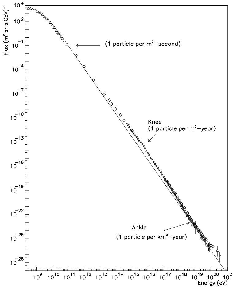
Abbildung 1.1: Das Energiespektrum der kosmischen Strahlung, das sich über einen Bereich von 15 Dekaden erstreckt. Für den Energiebereich unterhalb des „Knies“ (zwischen 10^{15} eV und 10^{16} eV) werden Supernova-Überreste als Beschleuniger angenommen. Aus [Aug96].
