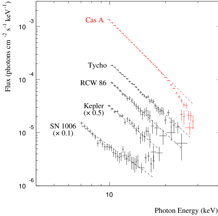
Abbildung 11.3: PCA-Spektren des RXTE-Satelliten von einigen Supernova-Überresten. Die Spektren lassen sich durch Potenzgesetze beschreiben und werden üblicherweise als Indikatoren für nicht-thermische Elektronen mit Energien bis in den TeV-Bereich gewertet. Aus [PAH99].
