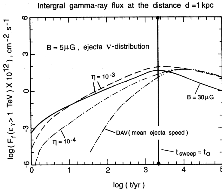
Abbildung 1.3: Simulation der zeitlichen Entwicklung der TeV- \gamma -Emission eines Supernova-Überrestes. Die stärkste Emission wird nach Erreichen der Sedov-Phase erwartet. Aus [Völ97].
