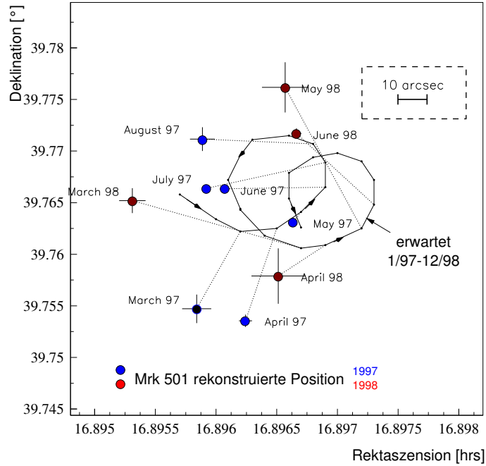
Abbildung 9.2: Rekonstruierte Position von Mrk 501 in Himmelskoordinaten. Das Bild stammt aus einer etwas älteren Analyse, die Rektaszension ist im Gegensatz zur üblichen Methode aufsteigend aufgetragen. Die Daten sind nicht auf eine gemeinsame Epoche korrigiert. Die Punkte mit Fehlerbalken geben die rekonstruierten TeV-Positionen wieder; die Punkte, die durch eine durchgezogene Linie verbunden sind, zeigen die erwartete Röntgenposition. Der systematische Ausrichtungsfehler beträgt 25'' pro Achse, das entspricht einem mittleren erwarteten Ausrichtungsfehler von \sigma = 35'' .
