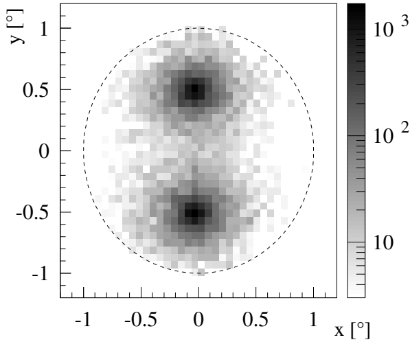
Abbildung 9.13: Signaldichtefunktion P_s unter der Annahme, daß alle in der Maximum-Likelihood-Analyse verwendeten Ereignisse des Cas A-Datensatzes \gamma -Ereignisse von der Quelle sind. Hiermit wird die ausreichende Normierung von P_s untersucht. Die Farbskala wurde so gewählt, daß Einträge oberhalb eines Promilles vom Maximum der Verteilung sichtbar werden.
