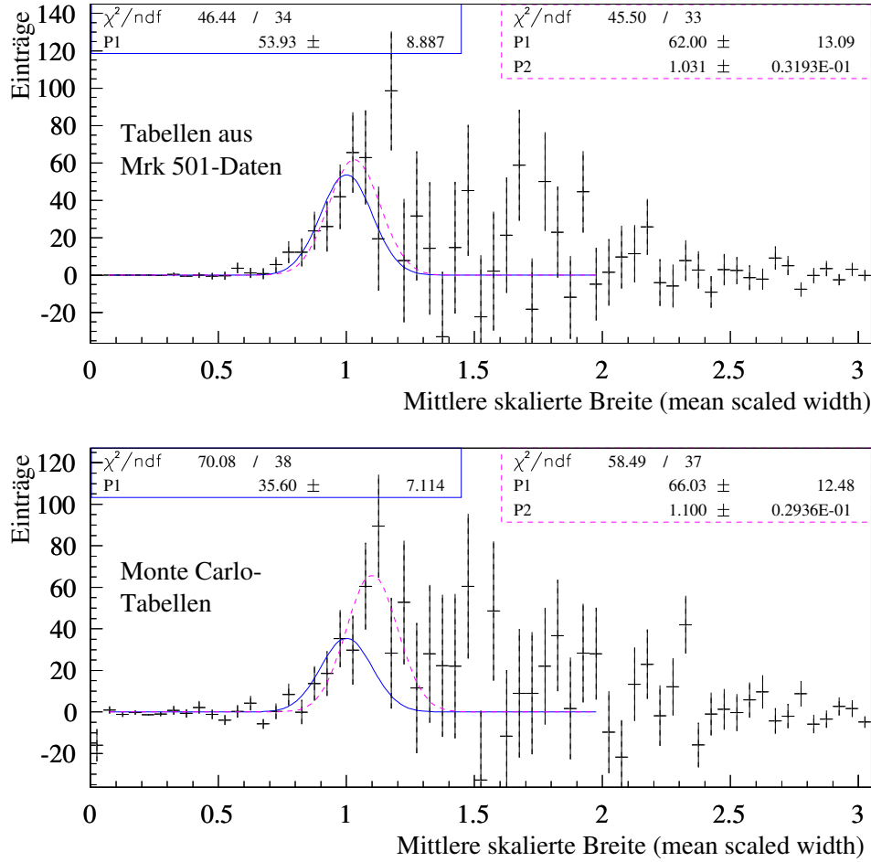
Abbildung 7.13: Mittlere skalierte Breite des Cas A- \gamma -Überschusses unter Verwendung der \gamma -Erwartungswerte, die aus den Mrk 501-Daten gewonnen wurden (oben). An die Verteilung wurde eine Gaußkurve der Breite \sigma = 0.1 angepaßt, wobei der Schwerpunkt der Verteilung \langle \tilde{w} \rangle_0 einmal fixiert wurde (durchgezogene Kurve) und einmal freigelassen wurde (gestrichelte Kurve). Das \chi^2 beider Verteilungen ist akzeptabel, der Schwerpunkt wird nur eine Standardabweichung neben dem Erwartungswert rekonstruiert; die Verteilung ist mit der \gamma -Erwartung gut verträglich. Unten ist derselbe Test unter Verwendung der Monte Carlo-Tabellen für die width -Erwartungswerte gezeigt. Man erkennt, daß man in diesem Fall deutlich unbefriedigendere Testergebnisse erhalten hätte.
