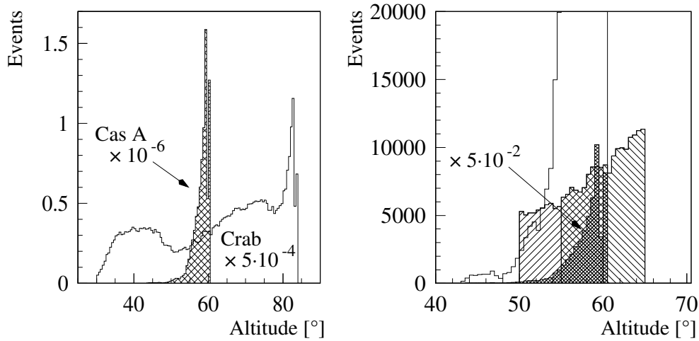
Abbildung 10.5: Zenitwinkelverteilung aller (Untergrund-)Ereignisse des Cas A- und des Krebsnebel Datensatzes im Vergleich. Links sind die vollen Datensätze gezeigt, rechts ist der Krebsnebel Datensatz auf den Zenitwinkelbereich zwischen 25^\circ und 40^\circ eingeschränkt und in 5^\circ -Schritten durch unterschiedliche Schraffierung markiert. Bei einer Gewichtung der Krebsnebel Daten entsprechend der Cas A-Zenitwinkelverteilung würde der statistische Fehler der Krebsnebel- \gamma -Verteilungen zu einem signifikanten Beitrag zum Fehler der Cas A-Spektrumsbestimmung führen. Daher werden hierfür alle Krebsnebel Daten zwischen 25^\circ und 40^\circ verwendet. Der dadurch verursachte systematische Fehler wird durch einen Vergleich der Untergrundspektren abgeschätzt.
