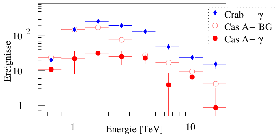
Abbildung 6.3: Vergleich der Rohspektren des Cas A- und des Referenzdatensatzes vom Krebsnebel. Die spektralen Verläufe der beiden \gamma -Spektren sind ähnlich. Aufgrund der zusätzlichen Kriterien der Ereignis Selektion bei der Bestimmung des Energiespektrums stehen nur etwa 60% der gesamten \gamma -Ereignisse zur Verfügung. Zusätzlich ist die Untergrunderwartung in den Cas A-Daten gezeigt; die Untergrunderwartung in den Krebsnebel Daten ist aufgrund der etwa 5-mal geringeren Beobachtungsdauer entsprechend kleiner. Der integrale TeV- \gamma -Fluß von Cas A beträgt ca. 3% des Krebsnebel flusses.
