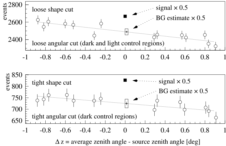
Abbildung 8.4: Ereigniszahlen in den Kontrollregionen des Cas A-Datensatzes, oben nach Anwendung lockerer Schnitte ( msw < 1.2, \theta^2 < 0.0225^\circ ), unten nach harten Schnitten ( msw < 1.1, \theta^2 < 0.0135^\circ ). Die Daten sind als Funktion des mittleren Zenitwinkels der jeweiligen Region relativ zum Zenitwinkel der Quellposition aufgetragen. Die offenen Symbole geben die Daten in den Untergrundkontrollregionen wieder; das kleine Kreuz zeigt ihren Mittelwert und damit den Untergrunderwartungswert in der Signalregion an, allerdings um einen Faktor 0.5 normiert, da die Signalregion zweifach gezählt wird. Der offene Kasten spiegelt die erwartete Untergrundstreuung wieder. Die gefüllten Symbole geben den Meßwert in der Signalregion wieder, ebenfalls um einen Faktor 0.5 normiert.
