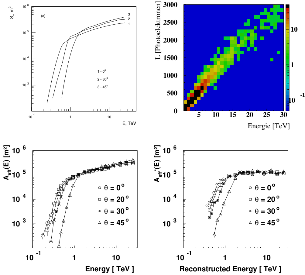
Abbildung 10.1: Ergebnisse der Schauer- und Detektorsimulationen zur Energie- und Spektrumsrekonstruktion für das HEGRA-Teleskopsystem. Oben links: Effektive Fläche S_\gamma = A_{\text{eff}} des Teleskopsystems für verschiedene Zenitwinkelbereiche. Die Funktion spiegelt ausschließlich die Triggerwahrscheinlichkeit für \gamma -Schauer einer bestimmten Energie wieder. Aus [KHA + 99]. Oben rechts: Abhängigkeit der Bildamplitude von der simulierten Schauerenergie. Der Zusammenhang wird genutzt, um aus der Bildamplitude in einem Teleskop die Energie zu rekonstruieren. Die gezeigte Abbildung gilt für einen Zenitwinkel von 20° und einen Abstand des Schauercores zum Teleskop von 80-100 m. Aus [Köh98]. Unten: Vergleich der reinen Ansprechwahrscheinlichkeit des Teleskopsystems (links) und der Korrekturfunktion, die zur Rekonstruktion des Spektrums genutzt wird (rechts). Zwei wesentliche Effekte bestimmen den Unterschied zwischen den Funktionen: Zum einen erfolgt eine Anhebung der effektiven Fläche zu kleinen Energien aufgrund der endlichen Auflösung der Energierekonstruktion (hier 20%). Zum anderen werden die Auswirkungen der Analyseschnitte sichtbar. Die Softwareschwelle von 40 Photoelektronen pro Bild bewirkt eine Anhebung der Energieschwelle; der Geometrieschnitt von 200 Metern Maximalabstand vom Schauercore zu einem Teleskop bewirkt eine Abflachung der effektiven Fläche zu hohen Energien. Aus [AAB + 99d].
