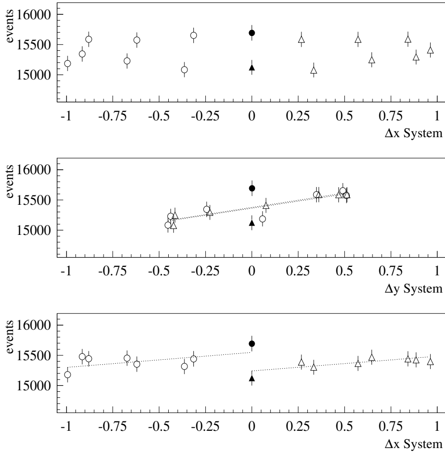
Abbildung 8.5: Ereigniszahlen in den Kontrollregionen des Cas A-Datensatzes ohne Anwendung eines Schauerformschnittes ( \theta < 0^\circ 15 ). Als horizontale Koordinate dienen hier die Systemgeometriechsen x_{\text{system}}/y_{\text{system}}/; x_{\text{system}} ist im Falle des Cas A-Datensatzes nahezu identisch mit dem Zenitwinkel. Die Daten wurden um die leicht unterschiedlichen Meßzeiten der Beobachtungen unter +0^\circ 5 und -0^\circ 5 Deklinationsabstand relativ zur Quelle korrigiert. Die offenen Symbole geben die Daten der Untergrundmessungen wieder; die Dreiecke bzw. Kreise stehen für die Beobachtungen unter den unterschiedlichen Vorzeichen des Deklinationsabstandes. Die gefüllten Symbole geben jeweils die Ereigniszahlen in der Signalregion an. Zu Details siehe Text.
