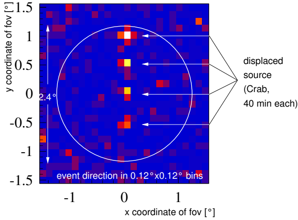
Abbildung 8.1: Für die Bestimmung der \gamma -Akzeptanz an verschiedenen Orten des Gesichtsfeldes gibt es (bisher) keine statistisch ausreichenden Beobachtungen. Simulationen ergeben eine auf 10% homogene Akzeptanz innerhalb eines Radius von 1^\circ . Die Abbildung links dient nur der Demonstration; in diesem Bild wurden die um die Bildfeldrotation korrigierten Gesichtsfelder von vier jeweils ca. 40-minütigen Beobachtungen überlagert, in denen sich der Krebsnebel an verschiedenen Positionen im Gesichtsfeld befand.
