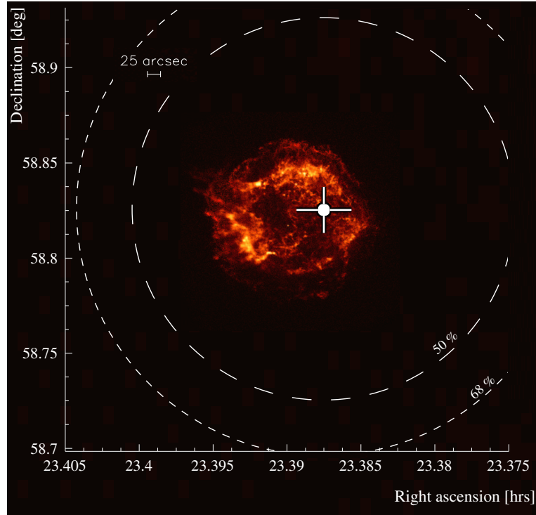
Abbildung 9.5: Der rekonstruierte Schwerpunkt der TeV- \gamma -Emission von Cas A im Vergleich zum Röntgenbild. Die gestrichelten Linien zeigen die 50%- bzw. 68%-Fehlerradien der Einzelereignisrekonstruktion an; diese wurden aus Krebsnebel- \gamma -Daten bestimmt. Im Rahmen des statistischen Fehlers ist die rekonstruierte TeV-Position von Cas A sowohl mit dem Mittelpunkt des SNR als auch mit einer Position auf der Schale konsistent.
