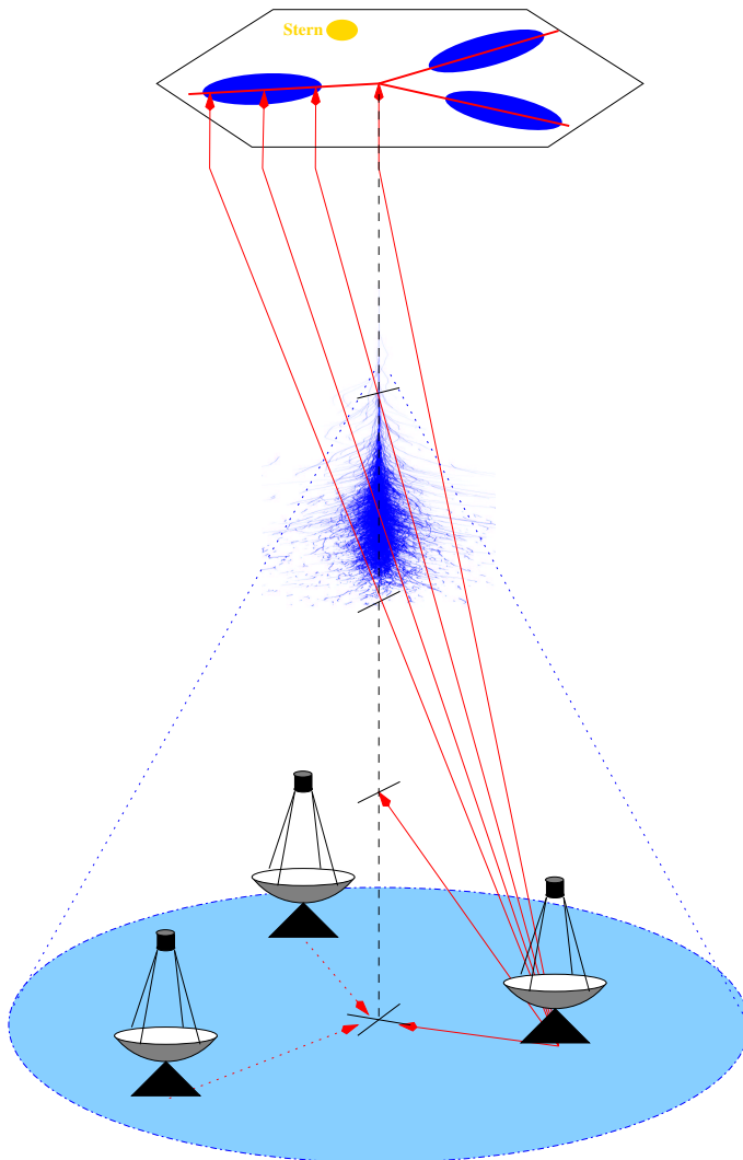
Abbildung 2.2: Schematische Darstellung der stereoskopischen Rekonstruktion von Luftschauern mittels eines Systems von abbildenden Cherenkov-Teleskopen. Die Teleskope sind winkellabbildend und parallel ausgerichtet, d.h. die Bildfelder am Himmel überlagern sich (im Bild oben durch das Hexagon angedeutet). In den Kameras entstehen Abbilder des an den Himmel projizierten Schauers. Die Herkunftsrichtung des Primärteilchens wird durch den Schnittpunkt der projizierten Schauerachsen bestimmt. Weiterhin wird durch das Schauerbild eine Ebene im Raum definiert, in der sowohl die Schauerachse als auch das jeweilige Teleskop liegen; diese Ebene ist im Bild für ein Teleskop durch die Vektorschar angedeutet. Durch den Kreuzungspunkt der von allen Teleskopen ausgehenden Vektoren, die am Erdboden entlanglaufen, wird der projizierte Schauerauftreffpunkt (Schauercore) bestimmt. Bei nicht-vertikaler Ausrichtung der Teleskope bleibt die Richtungsrekonstruktion unverändert; zur Bestimmung des Schauercores werden die Vektoren verwendet, die orthogonal zur Teleskopausrichtung stehen; diese werden in eine gemeinsame Ebene projiziert, wobei dann die bereits bestimmte Richtung der Schauerachse in geringem Maße eingeht.
