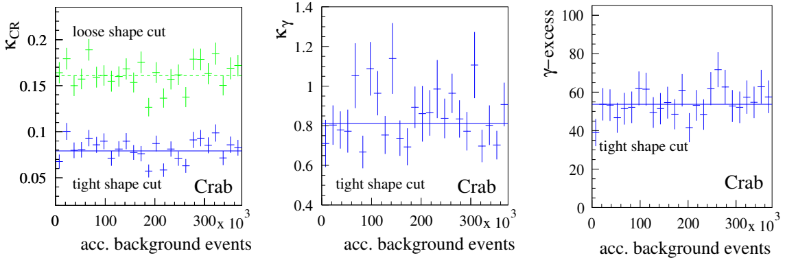
Abbildung 7.9: Dieselben Daten wie in Abb. 7.7, für den Krebsnebel Datensatz zwischen 25^\circ und 40^\circ Zenitwinkel.
