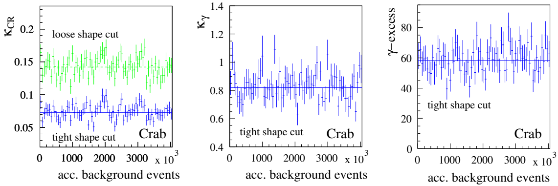
Abbildung 7.7: Verteilungen des Krebsnebel Datensatzes bei kleinen Zenitwinkeln ( 0^\circ - 25^\circ ) ohne schlechte Spiegeljustierung. Links: Untergrundunterdrückungseffizienz \kappa_{BG} des harten und des lockeren msw -Schnitts. Mitte: \gamma -Effizienz \kappa_\gamma des harten Schnitts. Rechts: \gamma -Ereignisrate nach Anwendung des harten Schnitts. Für alle Werte gilt ein Winkelschnitt von \theta^2 < 0.0135^\circ^2 .
