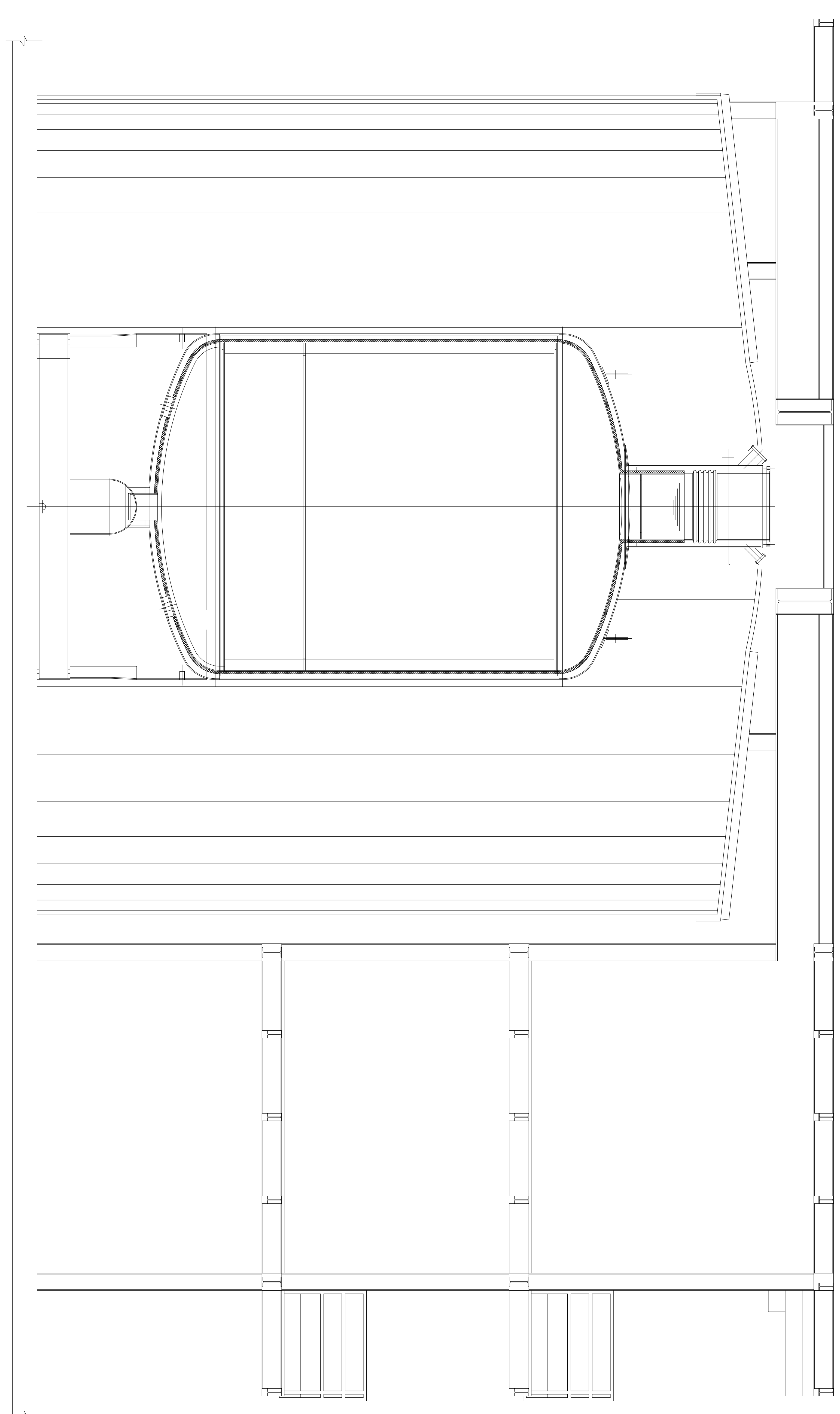
SEZIONE A-A
