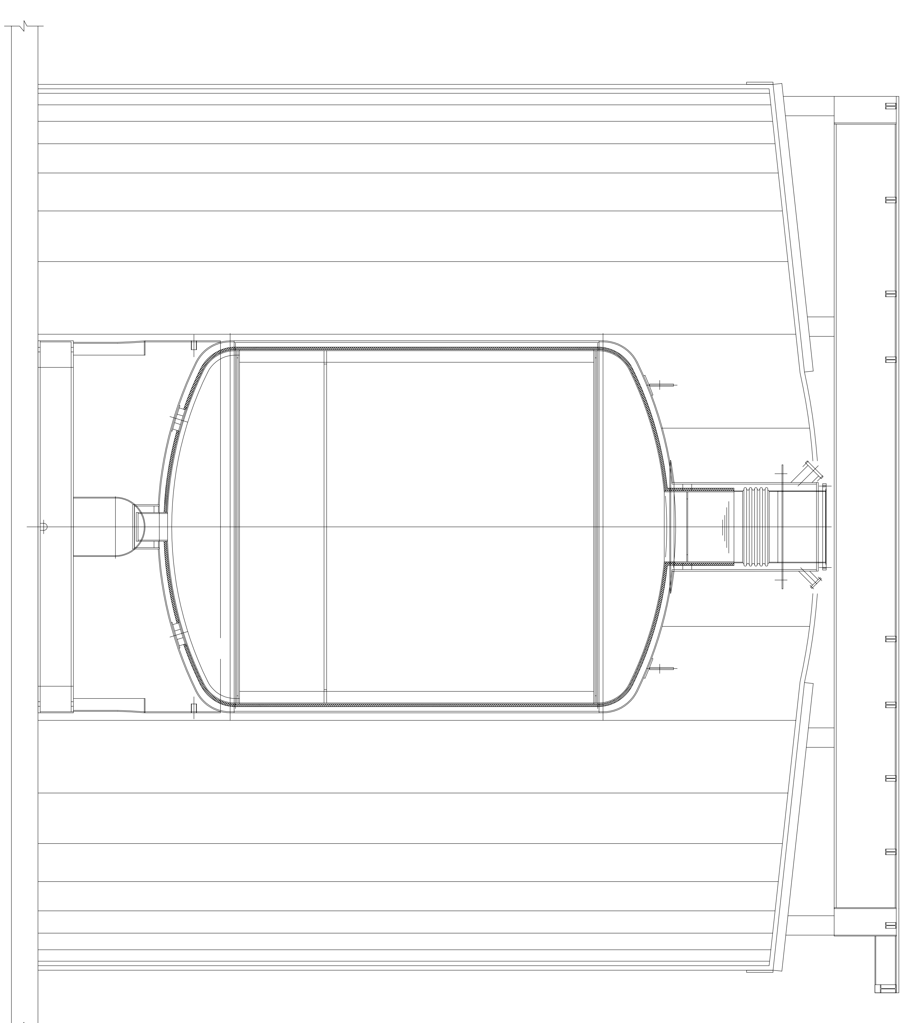
SEZIONE B-B
